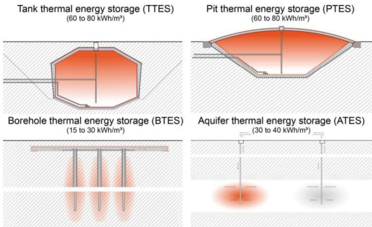
Slika 9. Tipovi sezonskih spremnika topline [17]
