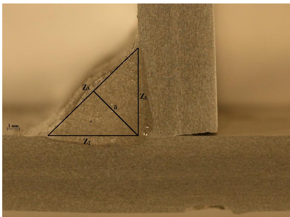
Slika 40. Geometrija zavara
