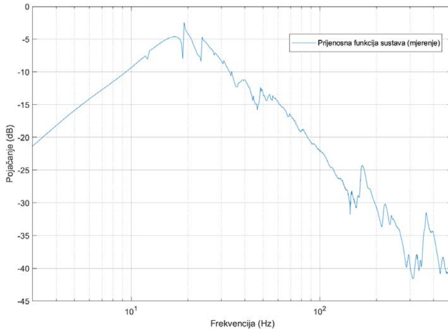
Slika 6.5 Pojačanje (mjerenje)
