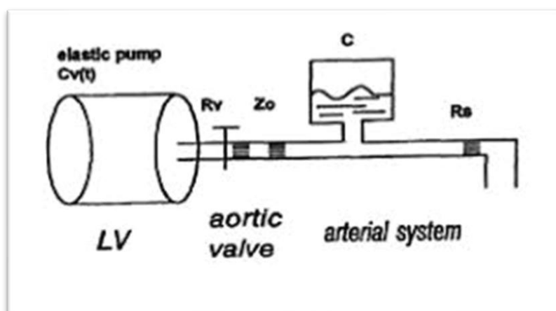
Slika 5.13. Hidraulička shema Windkessel modela s 3 elementa [17]
