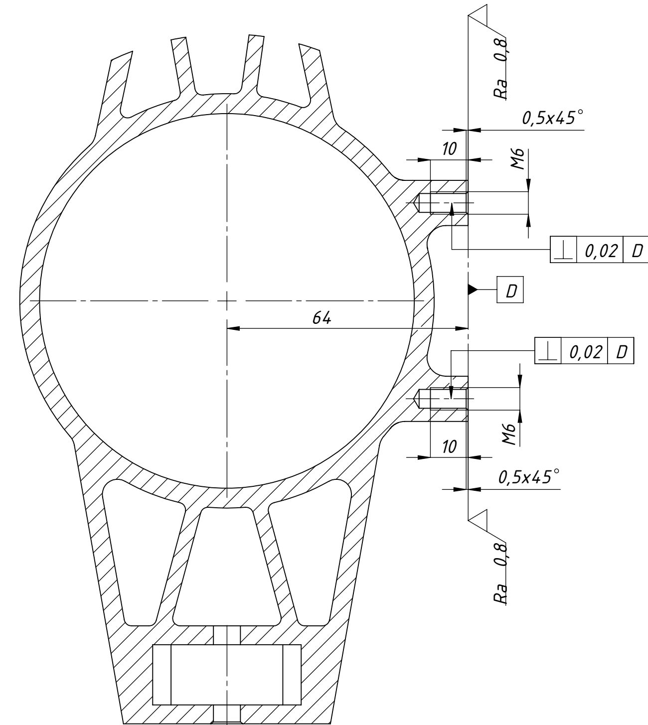
Presjek B-B Mjerilo M1 : 1
