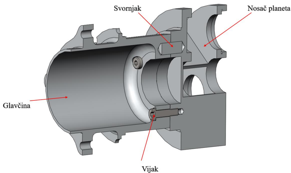
Slika 15. Spoj glavčine i nosača planeta
