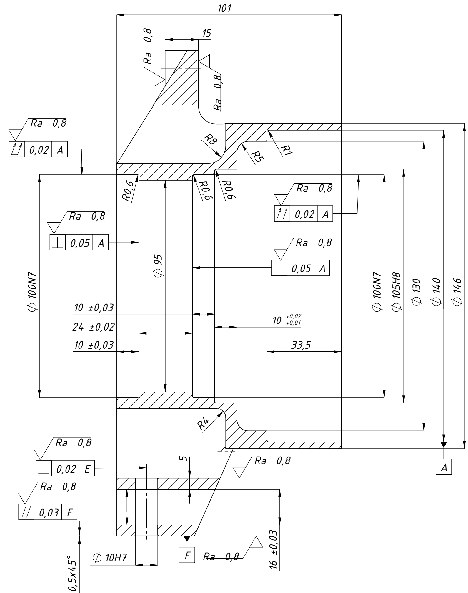
Presjek A-A Mjerilo M1 : 1
