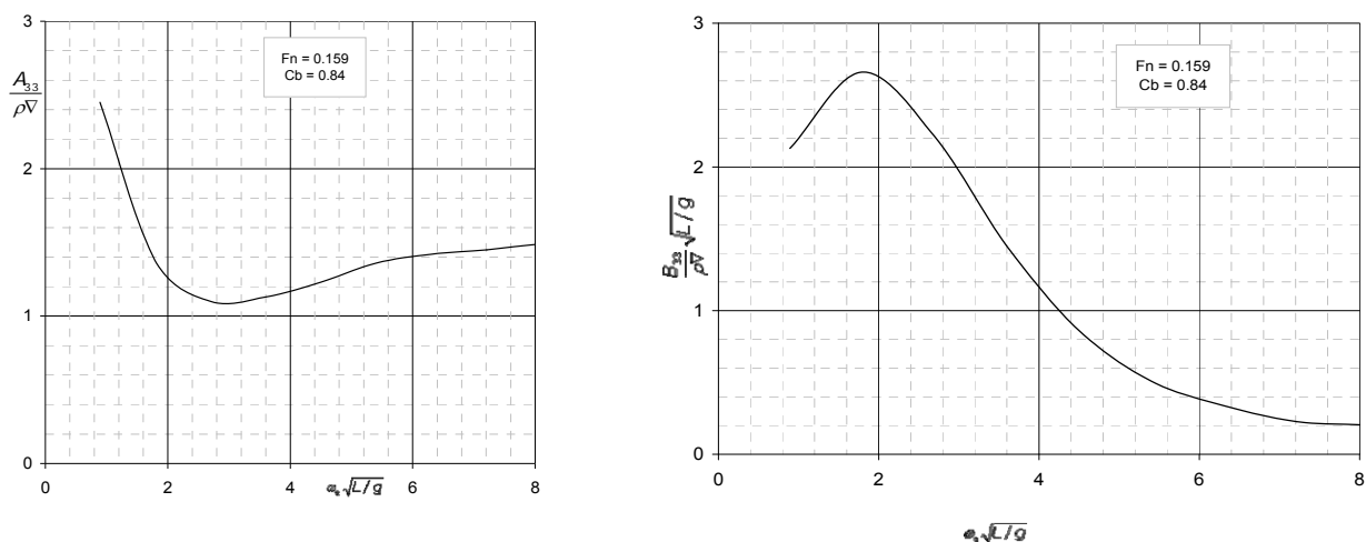
Dijagram 6.1 Hidrodinamički koeficijenti dodatne mase A_{33} koeficijenti prigušenja B_{33}
