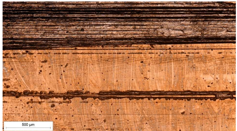
Slika 10.25. Alatni čelik K110 oznake D3 (TiN/TiBN prevlaka) na povećanju 50 puta
