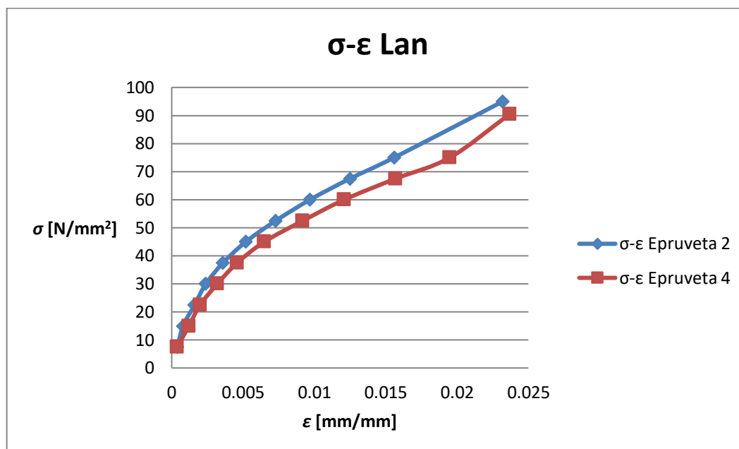
Slika 5.18. Dijagram „naprezanje - istežanje“ za lan
