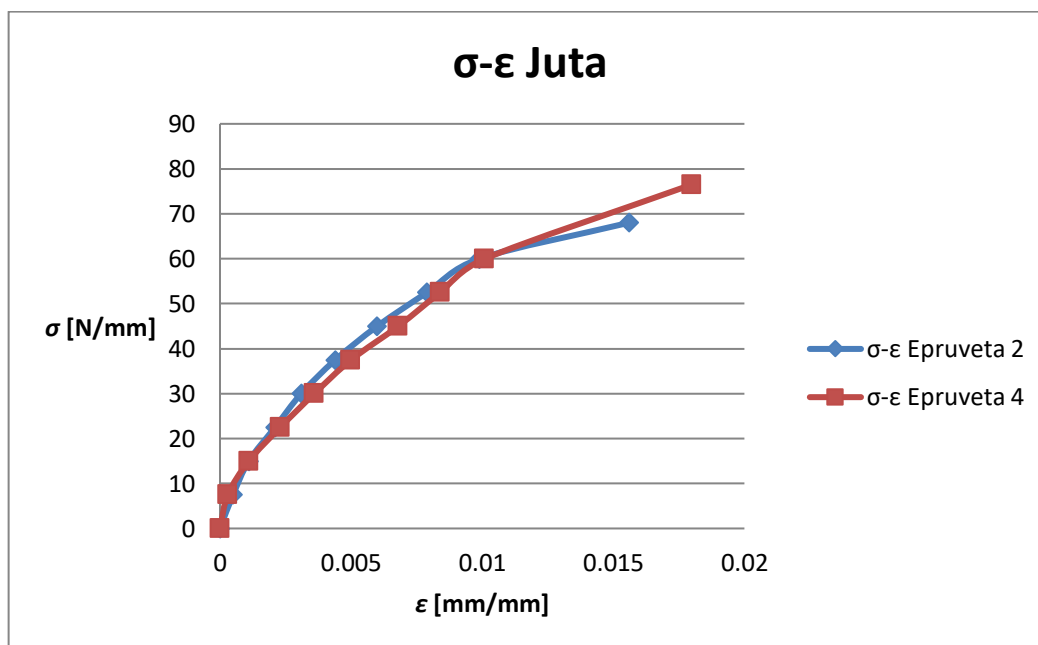
Slika 5.25 Dijagram „naprezanje - istežanje“ (juta)
