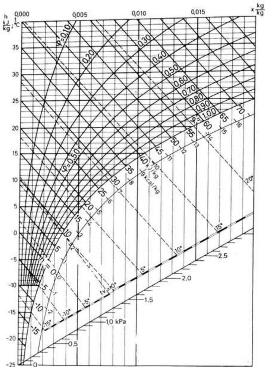
Slika 2. Mollierov dijagram
