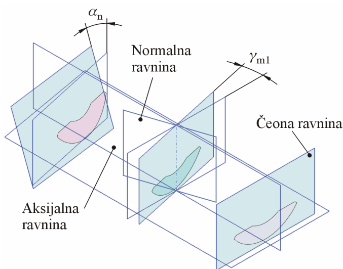
Slika 7.4 Projekcija površine zuba iz čeone ravnine
