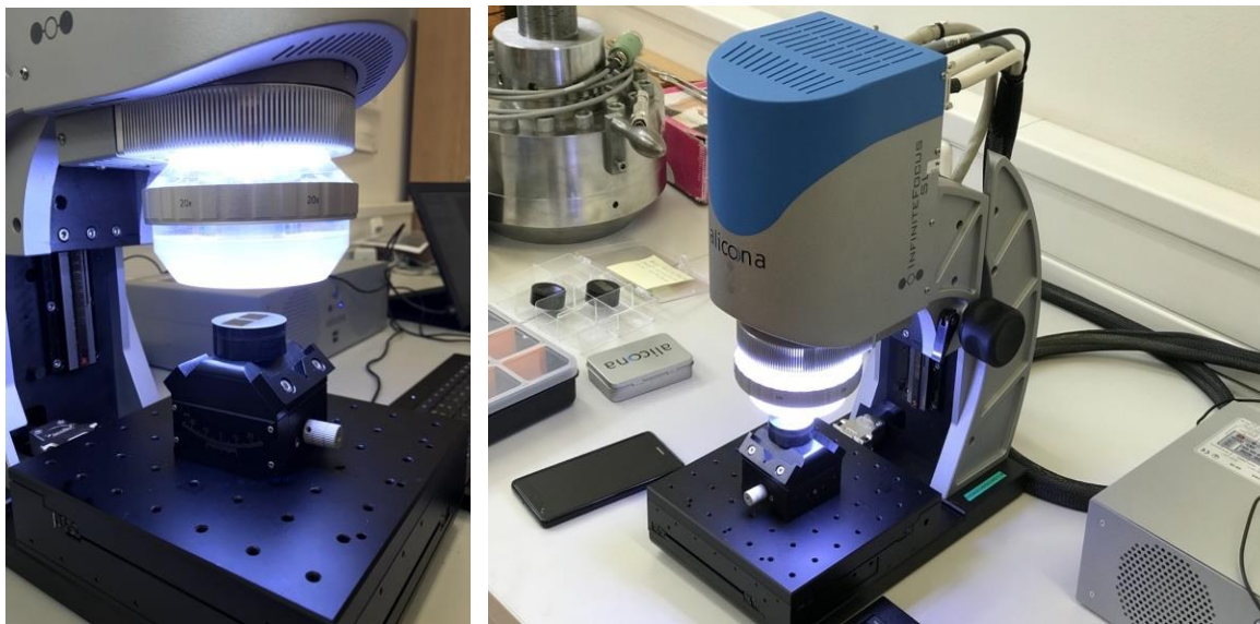
Slika 5.13 Ispitivanje površinske hrapavosti
