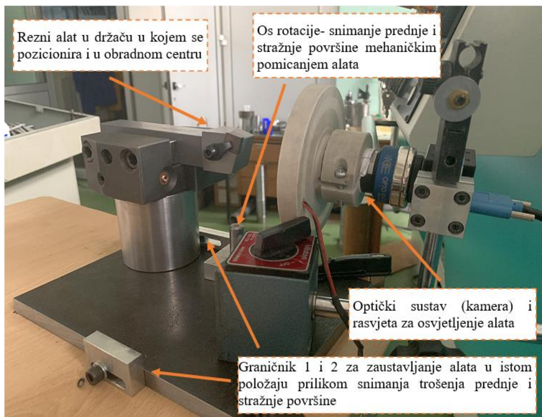
Slika 5.88 Prihvatna naprava za snimanje trošenja alata
