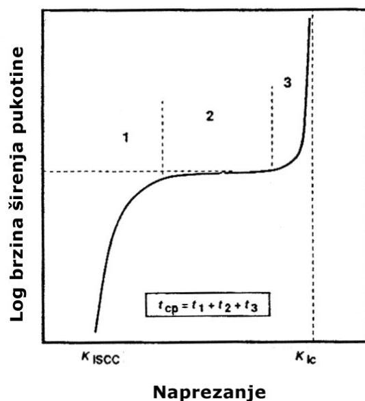
Slika 18: Test statički opterećenih neoštećenih uzoraka [3]
