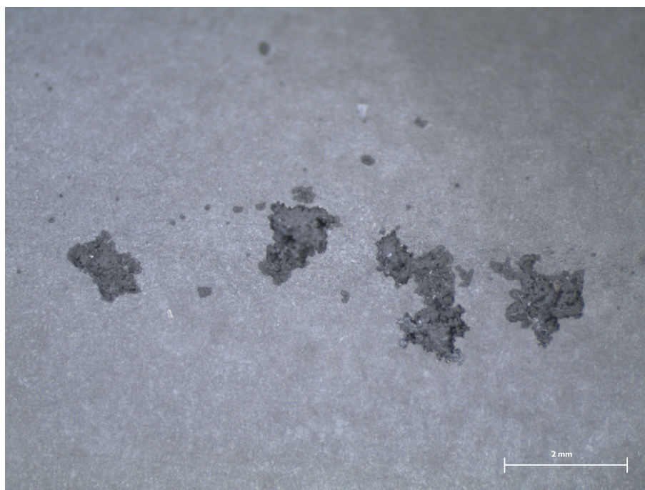
Slika 124: Stereomikroskopski snimak uzorka 21 (AISI 420) nakon ispitivanja – rupičasta korozija
