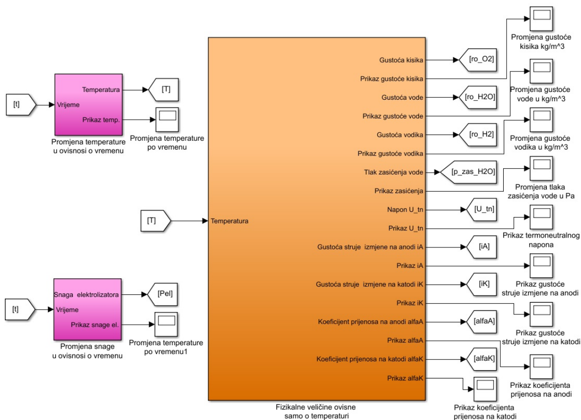
Slika 49. Simulink blokovi temperature, snage i parametara promjenjivih s temperaturom
