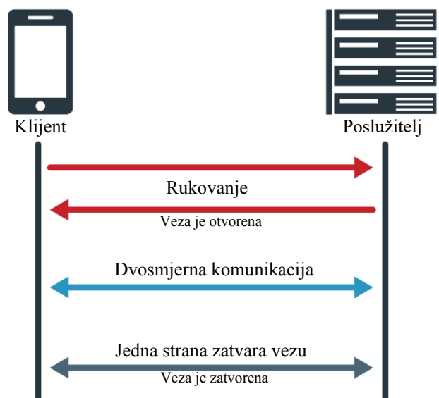
Slika 13. Princip rada WebSocket protokola [16]
