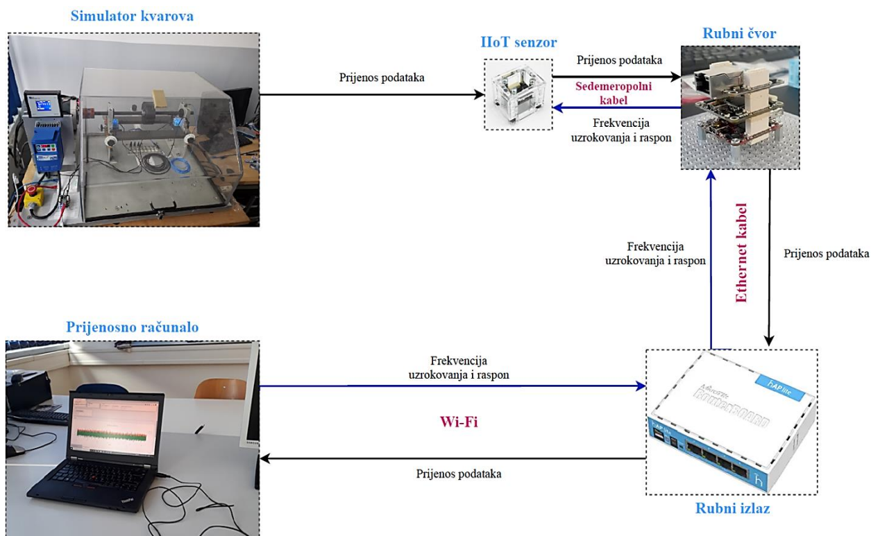
Slika 42. Shema simulacije rada sustava
