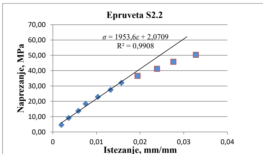
Slika 42. Krivulja naprezanje-istezanje za epruvetu S2.2
