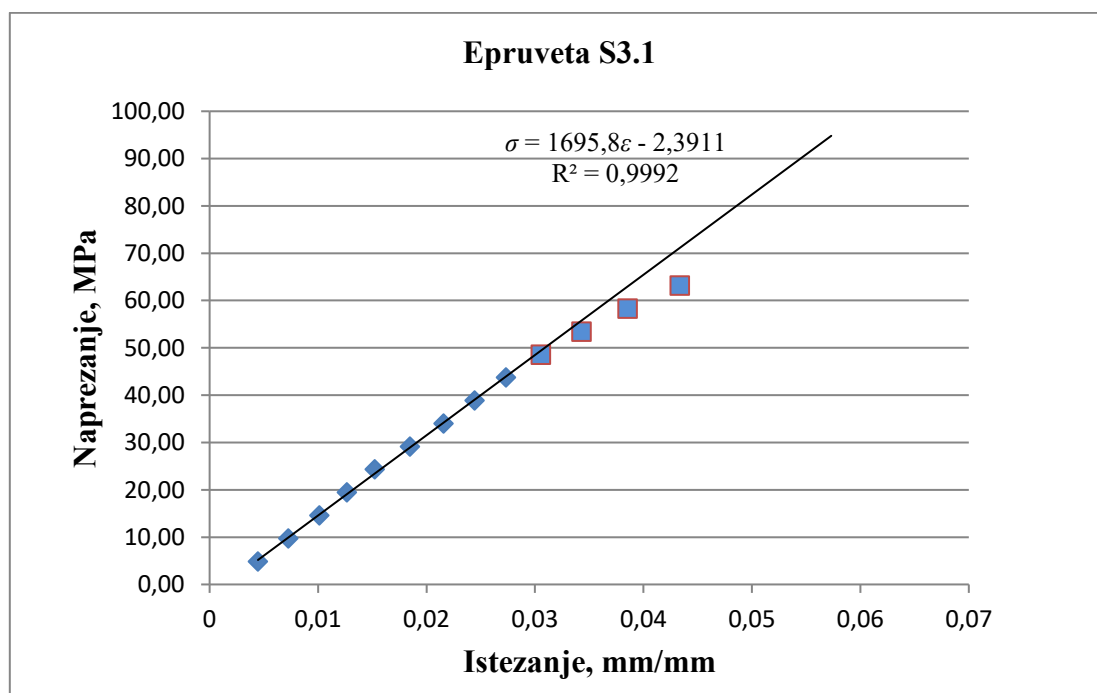
Slika 38. Krivulja naprezanje-istezanje za epruvetu S3.1
