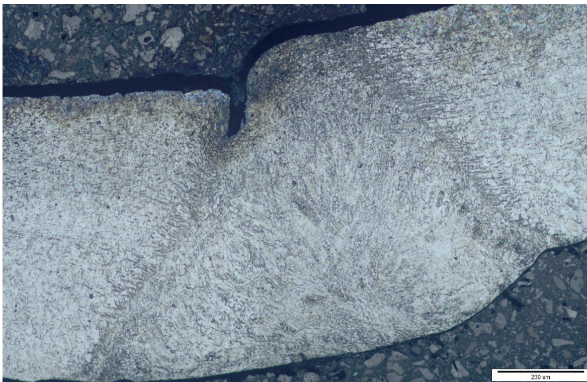
Slika 44. Makrostruktura zavarenog spoja
