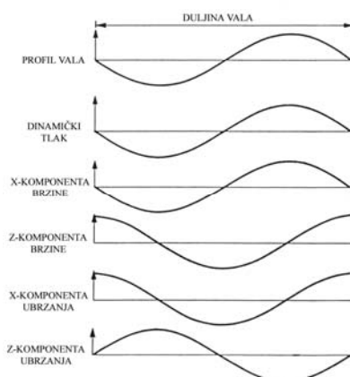
Slika 3.2 Profil vala te kinematičkih i dinamičkih značajki dobivenih linearnom teorijom [40]
