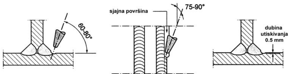
Slika 2.74 Naknadna obrada zavara čekićanjem [32]
