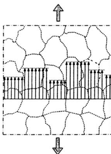
Slika 2.6 Pojednostavljeni prikaz nehomogene raspodjele napreznja na površini materijala [12]
