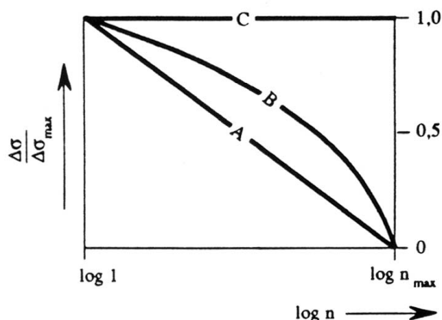
Slika 4.4 Uobičajeni spektri raspona napreznja (A) pravocrtni spektar (uobičajeni spektar raspona napreznja na valovima); (B) parabolni spektar (približna normalna razdioba raspona napreznja); (C) pravokutni spektar (uobičajeni spektar za raspone napreznja uslijed uzbude od motora, ili vijka) [69]
