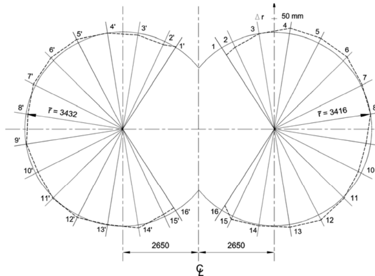
Slika 13-2 Odstupanje od idealnog oblika u ravnini poprečnog presjeka, \Delta r
