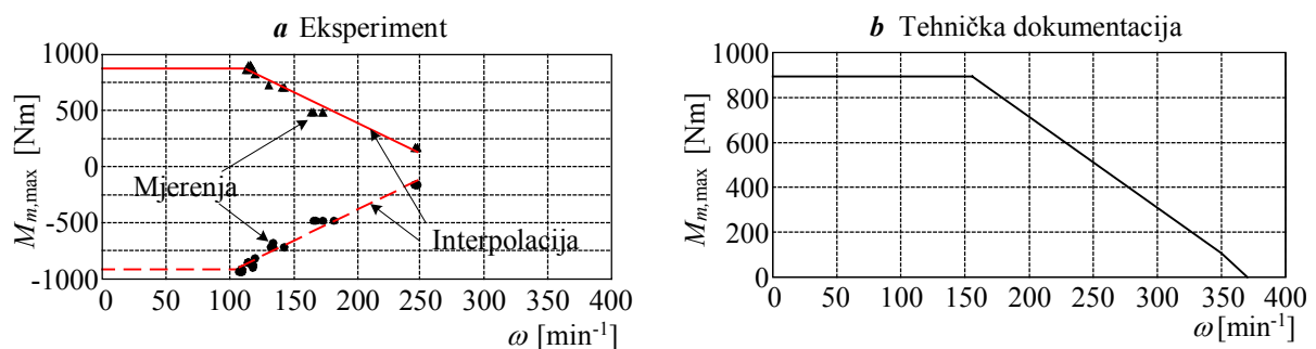
Slika 4.13. Maksimalni dostupni moment motora u ovisnosti o brzini vrtnje: procijenjen na vozilu (a) i iz tehničke dokumentacije proizvođača (b).
