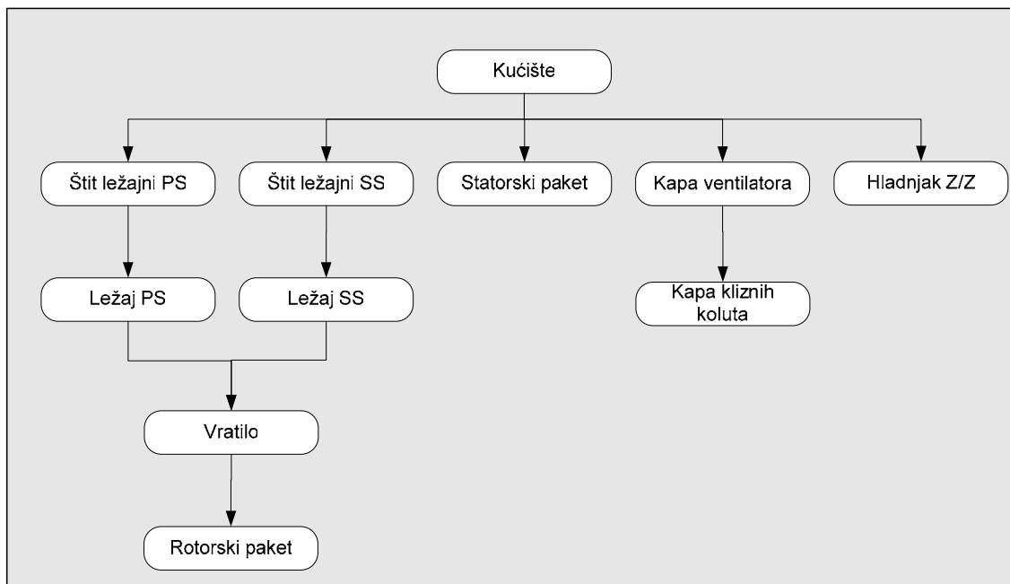
Slika 7 - 13: Hijerarhijska struktura osnovnih komponentata kod klizno-kolutnog asinkronog motora
