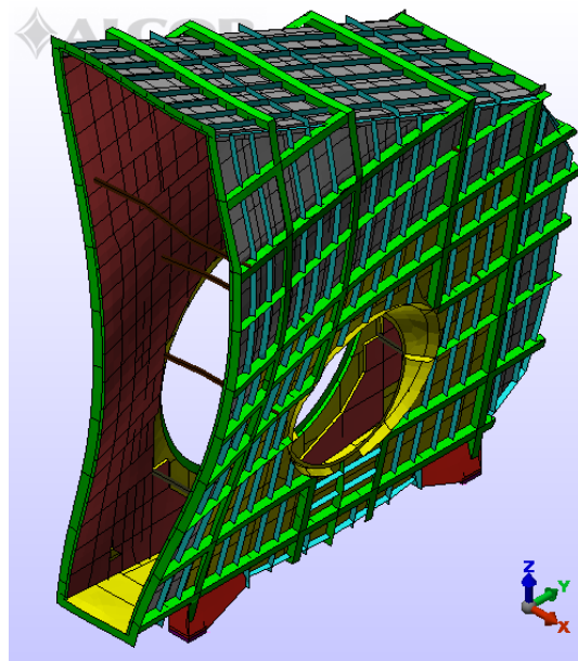
Slika 8.2.4 Drugi način vibriranja f_2 = 10,5 \text{ Hz}
