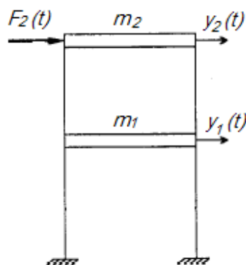
Slika 3.5.1 Ravninski model konstrukcije s dvije mase
