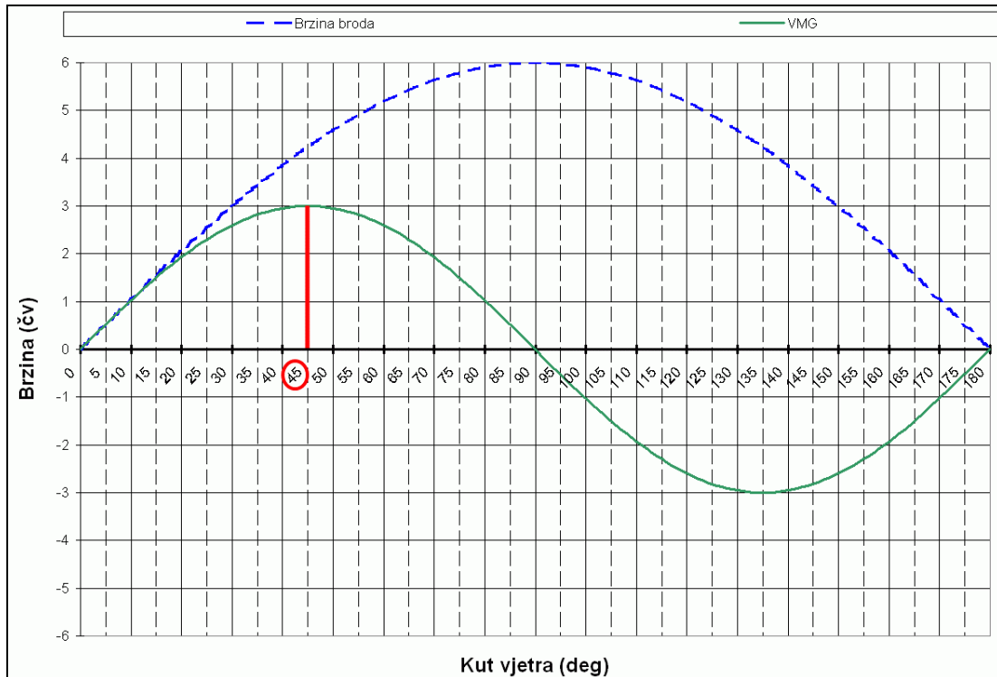
Slika 5-7: Prikaz brzine broda i VMG brzine za različite kutove vjetra
