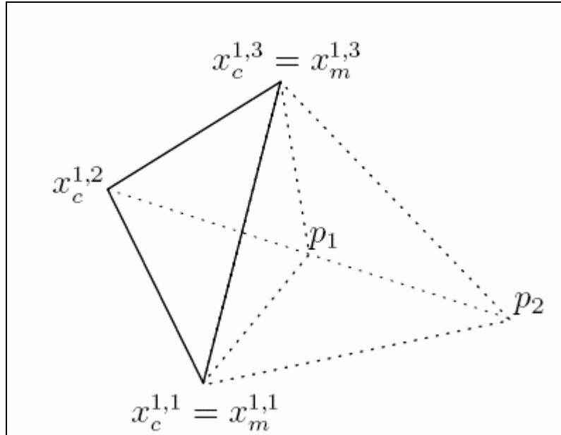
Slika 7-2: Primjer za SCGA mutaciju u dvije dimenzije
