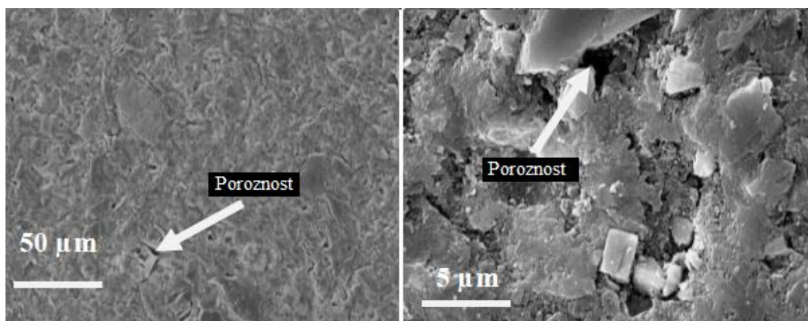
Slika 32. Mikrostruktura konvencionalno sinteriranog Al-SiC-TiC kompozita (uz različito povećanje) [41]
