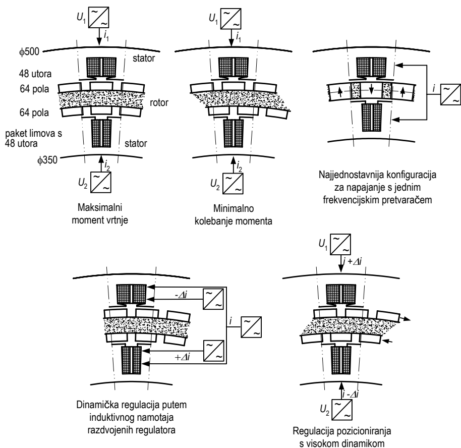
Slika 2.20 Varijacije povezivanja napajanja sa statorskim namotima za dupli stator u daljnjem razvoju PPSM-a
