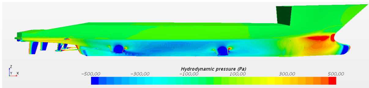
Slika 34. Raspodjela hidrodinamičkog tlaka na Modelu 2
