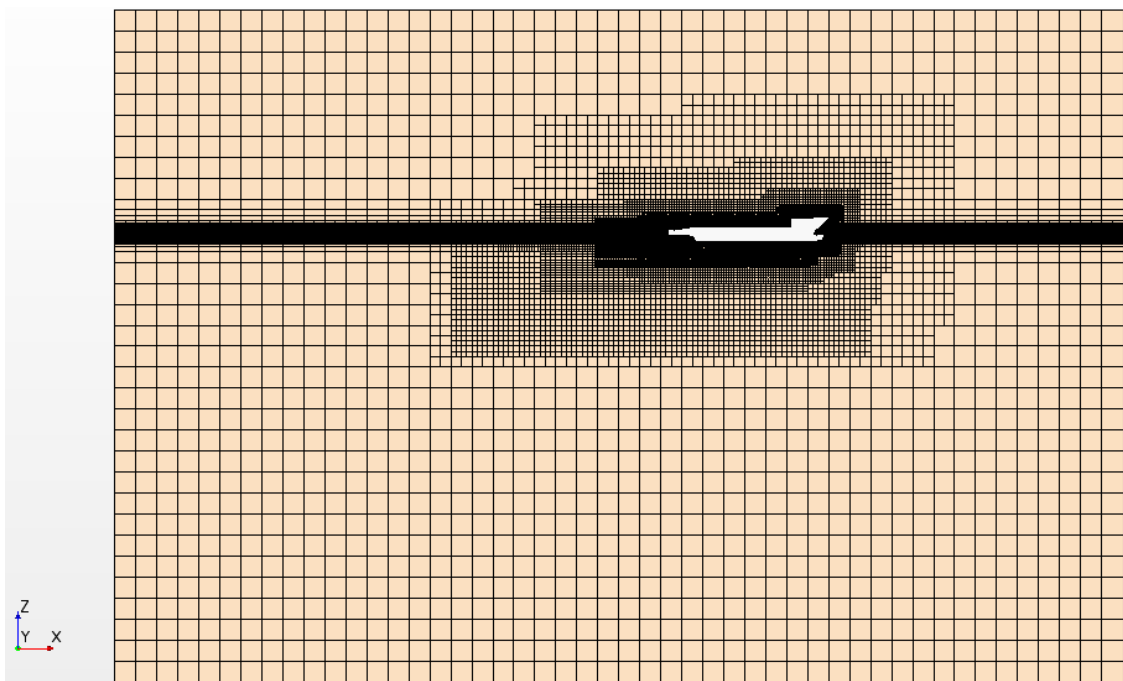
Slika 19. Diskretizacija geometrijske mreže Modela 2
