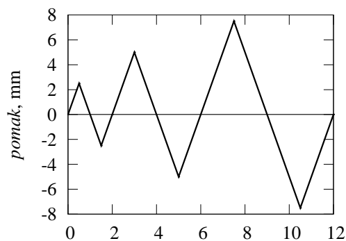
Slika 7.11: PRAVOKUTNA PLOČA: prikaz cikličkog opterećenja kvadratne ploče pomoću dijagrama koji daje ovisnost narinitog pomaka točke A o vremenu
