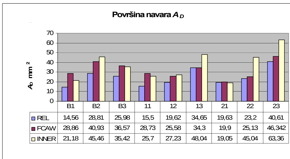
Slika 4.26 Površina navara A_D prema stanju pokusa
