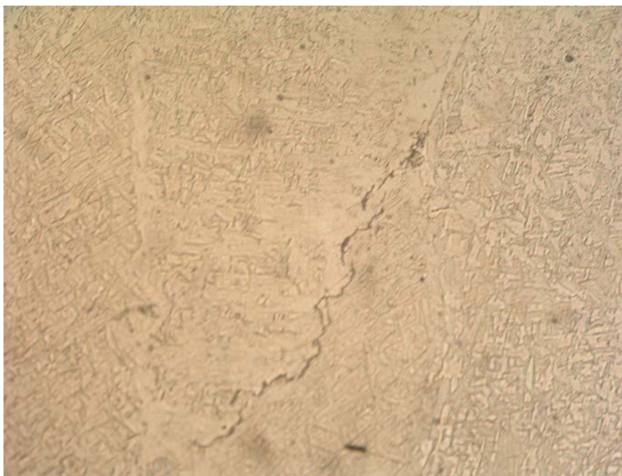
Slika 4.41 Pukotina u metalu zavora- uzorak F125, povećanje 200x
