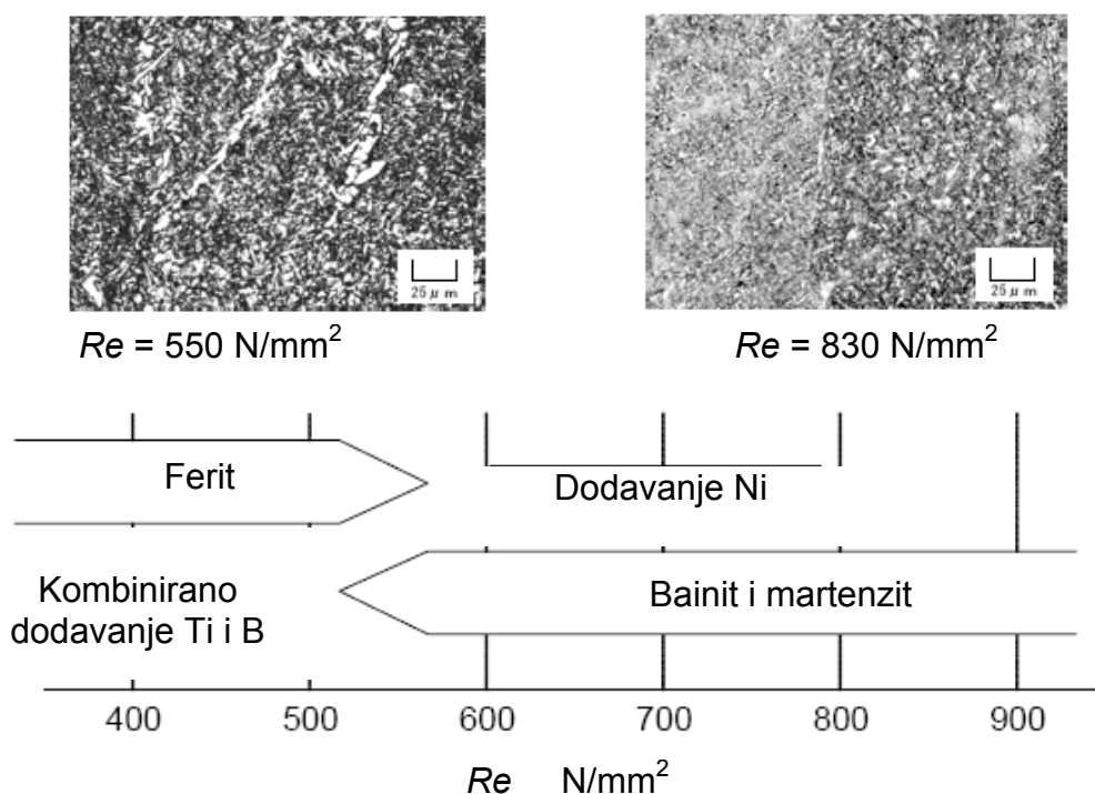
Slika 2.24 Metode legiranja za povećanje čvrstoće metala zavora [103]
