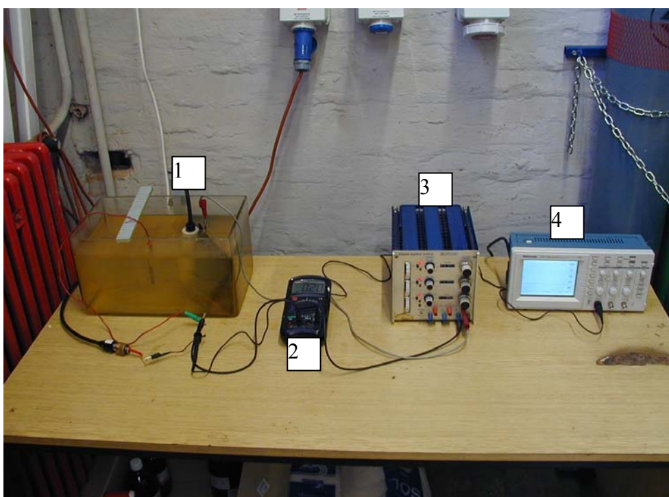
Slika 3.20 Sustav za simulaciju katodne zaštite
