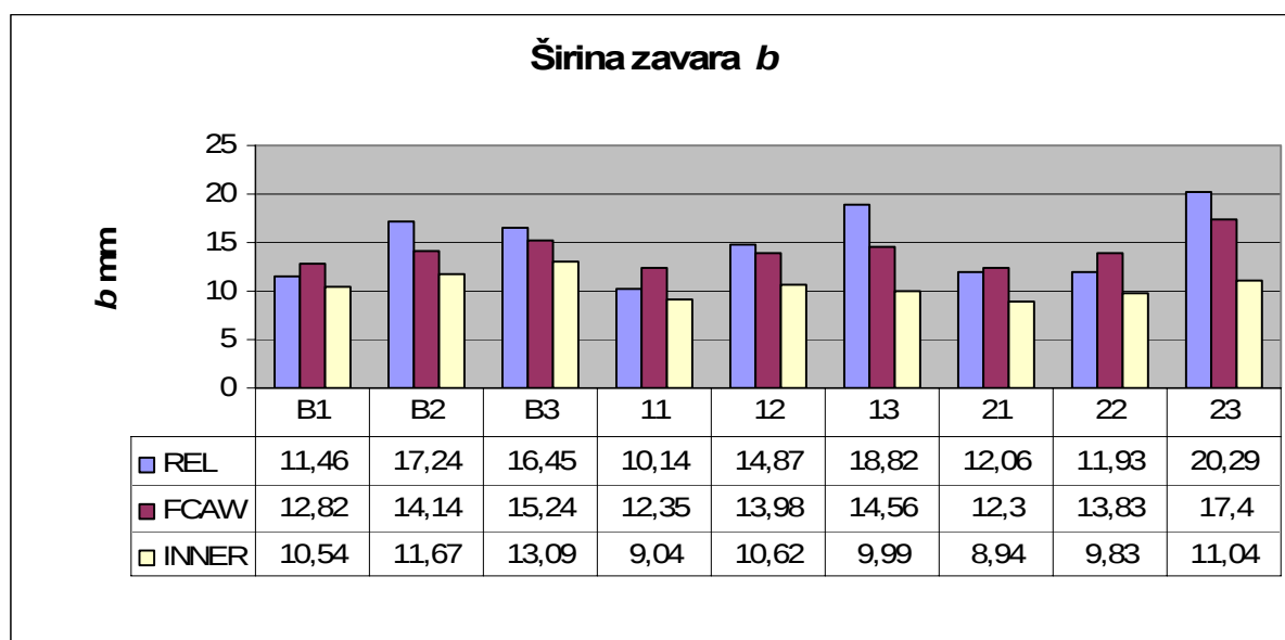
Slika 4.21 Širine zavora b prema stanju pokusa
