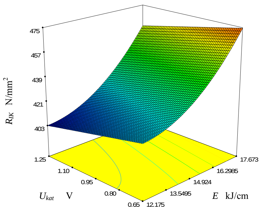
Slika 4.50 Odzivna površina R_{IK} za REL postupak zavarivanja
