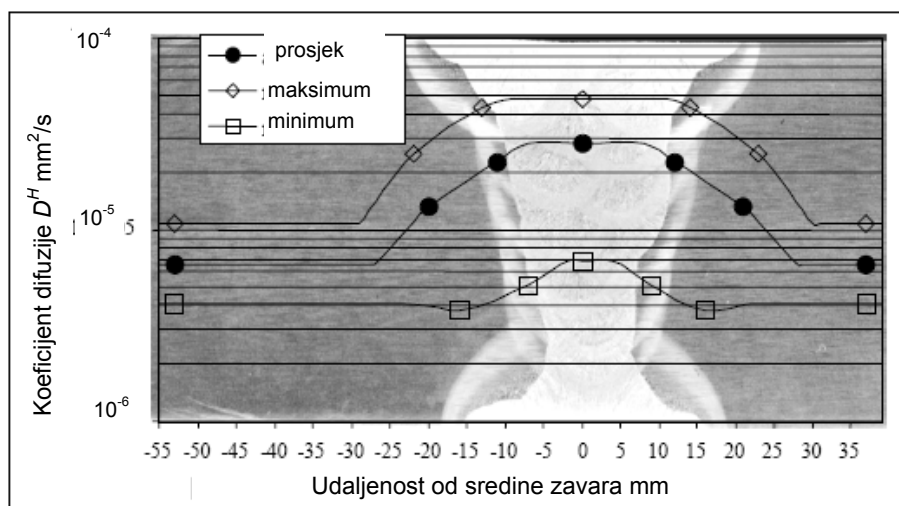
Slika 2.17 Ovisnost koeficijenta difuzije vodika o lokaciji u zavarenom spoju [63]
