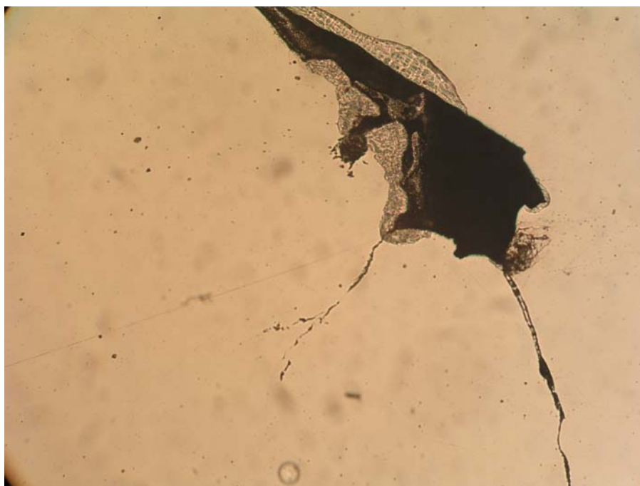
Slika 4.45 Propagacije pukotine iz uključka – uzorak F212, povećanje 200x, polirano stanje
