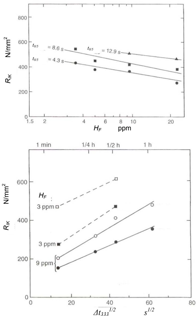
Slika 2.13 Ovisnost kritičnog Implant napreznja o koncentraciji i difuziji vodika za jedan mikrolegirani čelik (gornja slika) i jedan poboljšani čelik (donja slika) [31]
