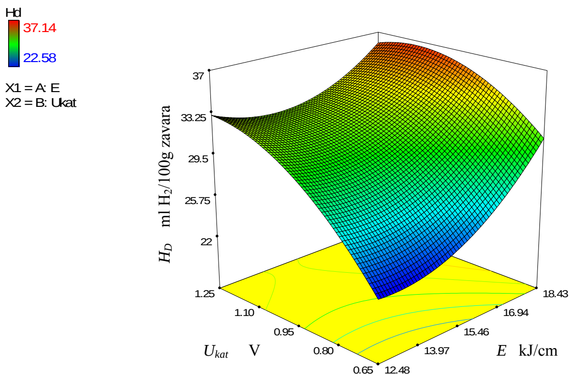
Slika 4.52 Odzivna površina H_D za zavarivanje praškom punjenom žicom u plinskoj zaštiti
