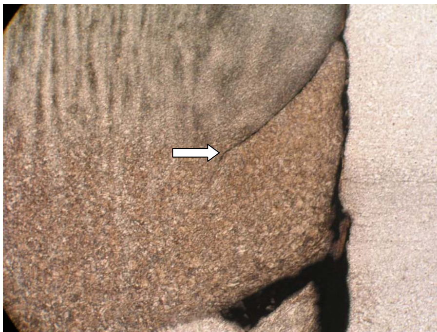
Slika 4.46 Inicijacija pukotine iz narezanog navoja na Implant epruveti-uzorak R215, povećanje 50x
