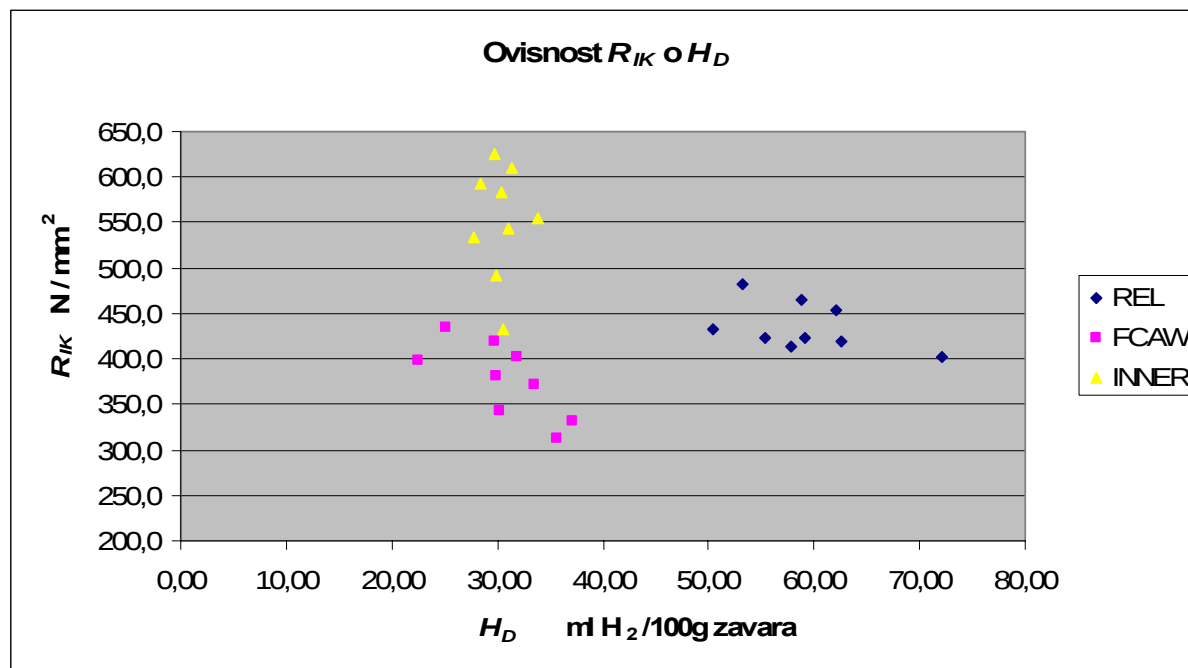
4.18 Prikaz ovisnosti kritičnog Implant naprezanja o količini difundiranog vodika
