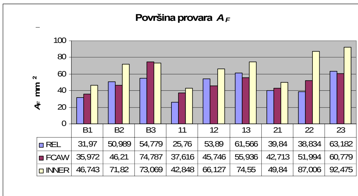
Slika 4.25 Površina provara A_F prema stanju pokusa
