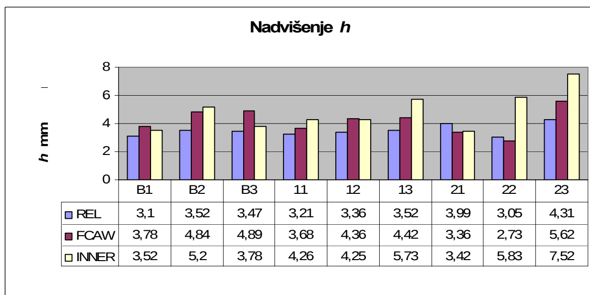
Slika 4.22 Nadvišenje zavora h prema stanju pokusa
