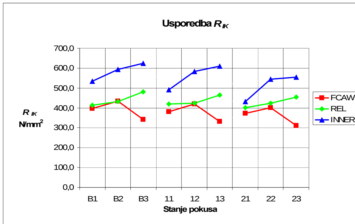
Slika 4.19 Usporedba kritičnog Implant naprezanja za postupke zavarivanja
