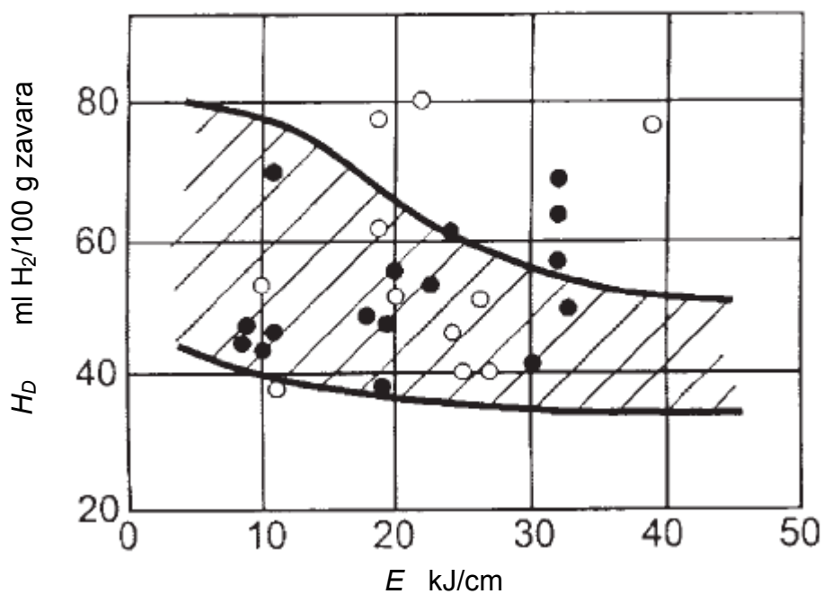
Slika 2.5 Utjecaj unosa topline na količinu difundiranog vodika pri mokrom podvodnom zavarivanju čelika St 37-2 ( I=180 do 250\text{A} , U=28 do 48\text{ V} , v_z=11 do 21\text{ cm/min} , ●-E4332, ○-E5122) [10]
