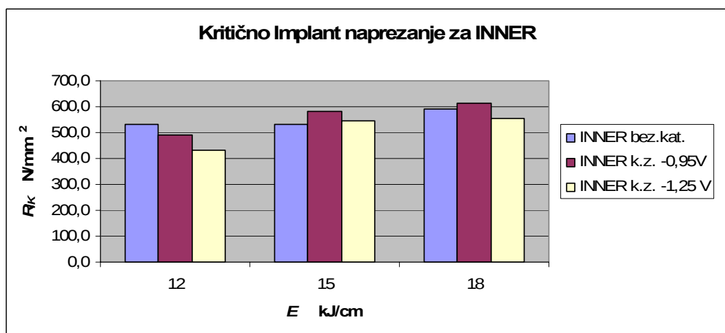
Slika 4.16 Prikaz rezultata R_{IK} za INNER
