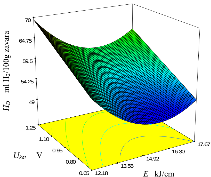
Slika 4.48 Odzivna površina H_D za REL postupak zavarivanja
