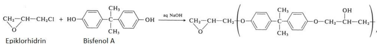
Slika 2.2. Kemijska reakcija nastanka Bisfenol A epoksidne smole [9]
