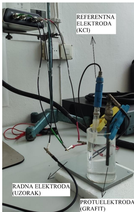
Slika 5.30. Pripremljeni uzorak prije početka mjerenja EIS-a
