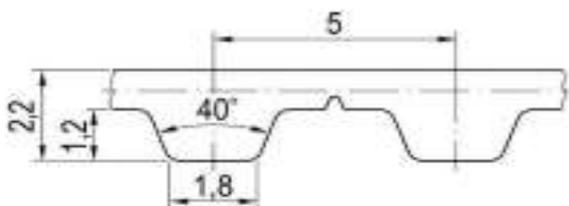
Slika 69. Profil remena [26]
