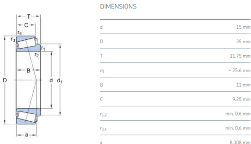
Slika 57. Dimenzije ležaja 30202
