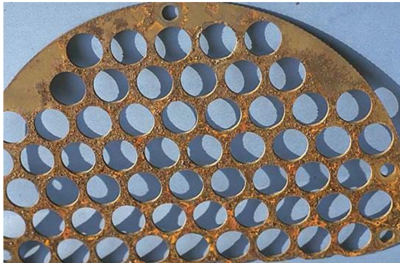
Slika 2.1. Korozija čelične pregrade u izmjenjivaču topline [5]
