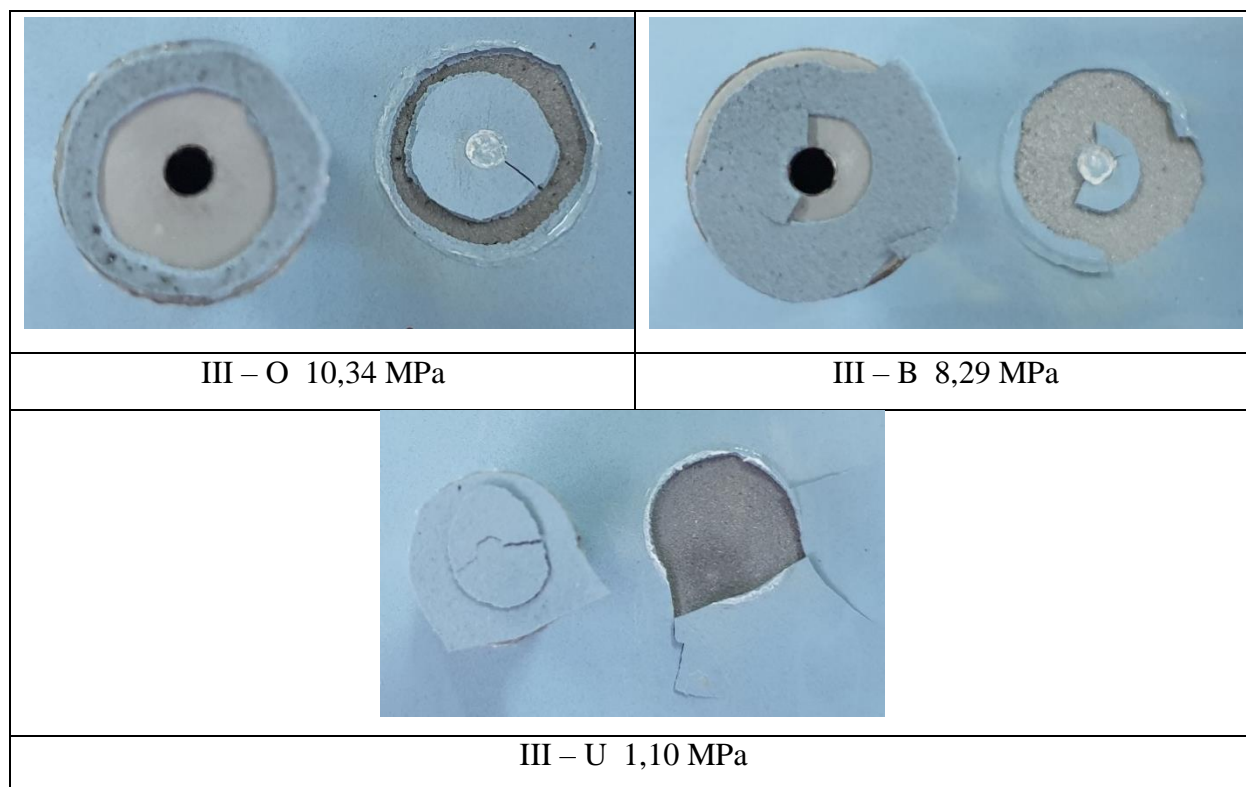
Slika 7.49. Rezultati Pull – off ispitivanja nakon vlažne komore
