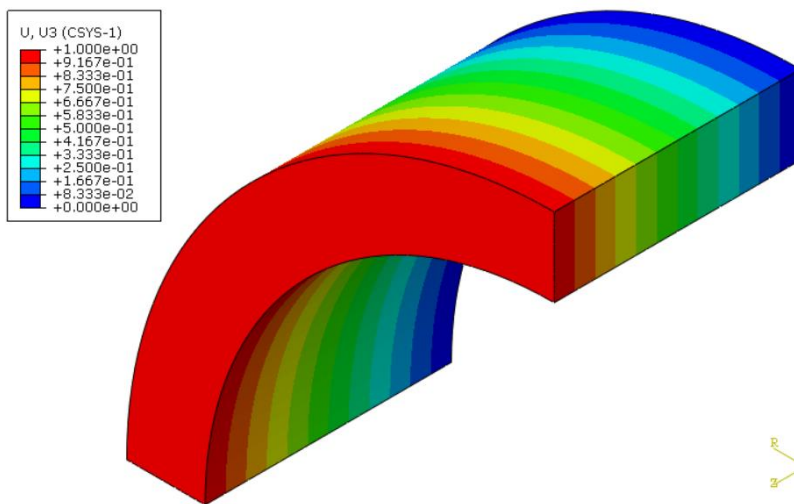
Slika 31. Pomak u aksijalnom smjeru - Mooney-Rivlin materijalni model
