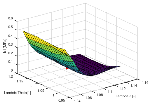
Slika 53. Utjecaj promjene vrijednosti \lambda_z i \lambda_\theta na materijalni parametar k_1
