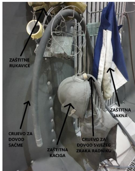
Slika 28. Kabina za sačmarenje u AKZ odjelu tvrtke Končar MK (lijevo) i oprema za sačmarenje (lijevo)
