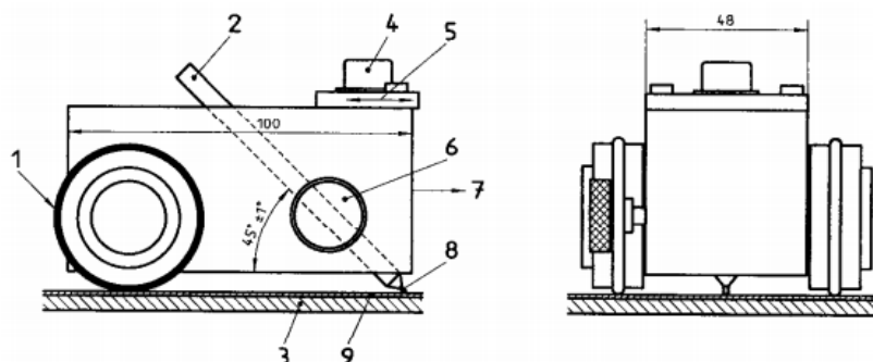
Slika 51. Uređaj za ispitivanje tvrdoće premaza olovkama prema normi HRN EN ISO 15184
