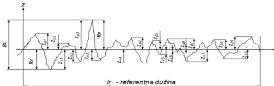
Slika 6. R_p , R_v i R_z parametri [1]
