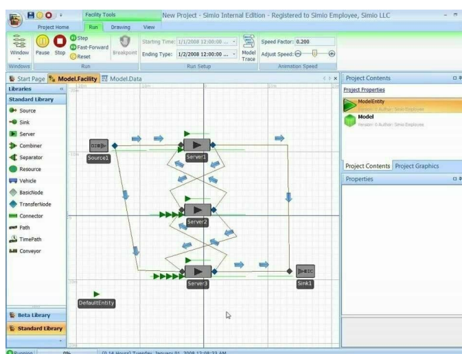
Slika 33 Sučelje Simio [18]
