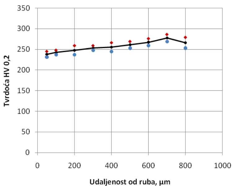
Slika 40. Raspored tvrdoće po poprečnom presjeku ispitnog uzorka od čelika C45 obrađenog postupkom vanadiranja u solnoj kupci
