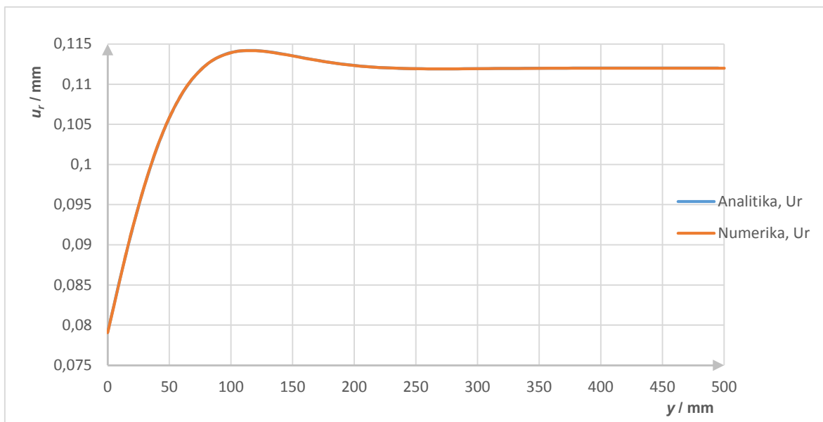
Slika 58. Raspodjela radijalnog pomaka cilindrične ljsuske
