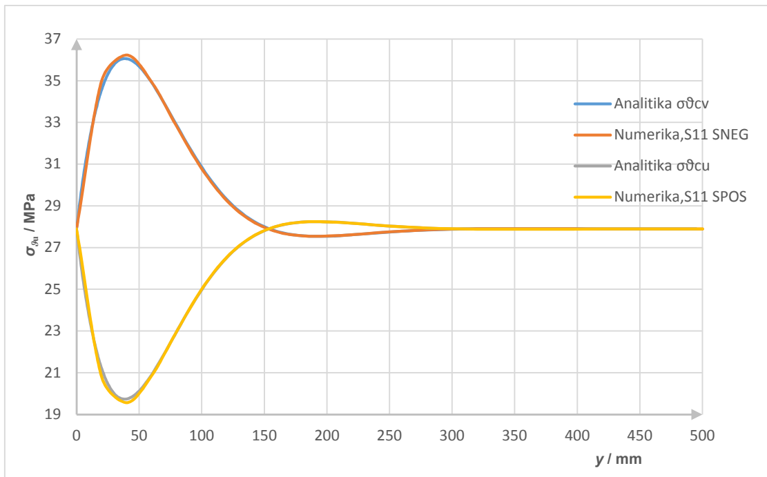
Slika 60. Raspodjela meridijalnog napreznja duž unutrašnjeg ruba cilindrične ljuske
