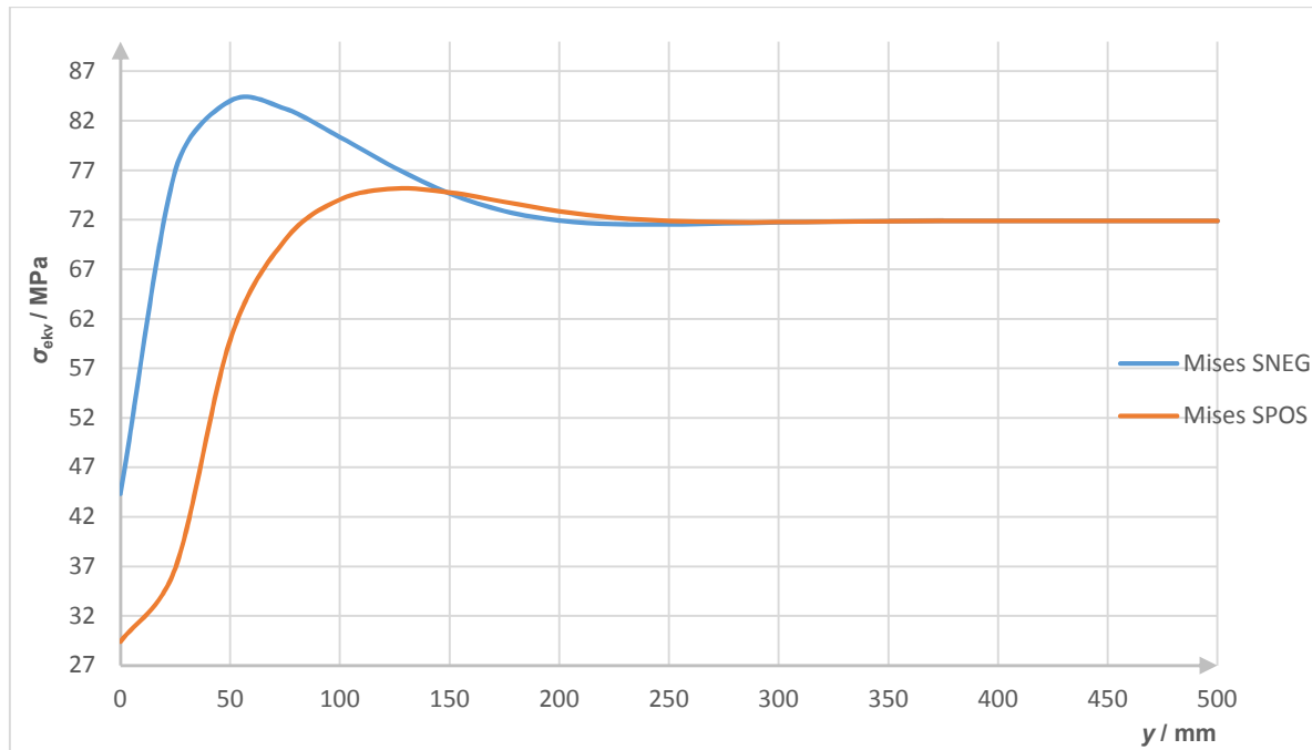
Slika 85. Raspodjela ekvivalentnog naprezanja duž vanjskog i unutarnjeg ruba cilindrične ljsuke - tlačna proba
