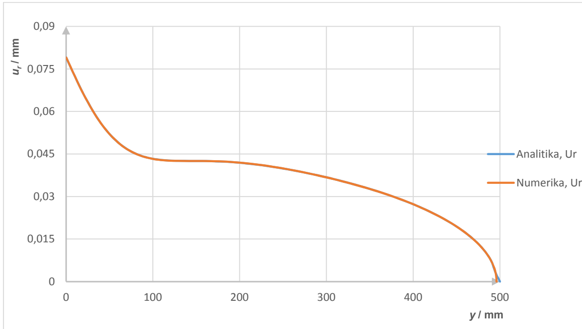
Slika 57. Raspodjela radijalnog pomaka sferne ljsuske
