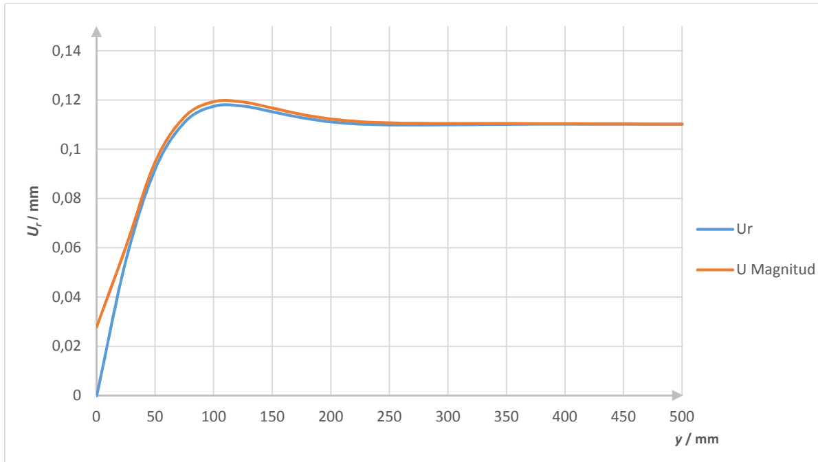
Slika 72. Raspodjela radijalnog pomaka cilindrične ljuste - radno opterećenje
