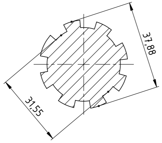
PRESJEK B-B 1 : 1
