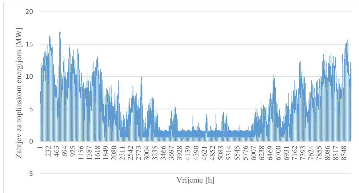
Slika 9. Potreba za toplinskom energijom
