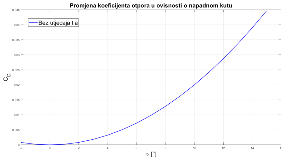
Slika 4 Promjena koeficijenta otpora C_D u ovisnosti o napadnom kutu \alpha bez utjecaja tla
