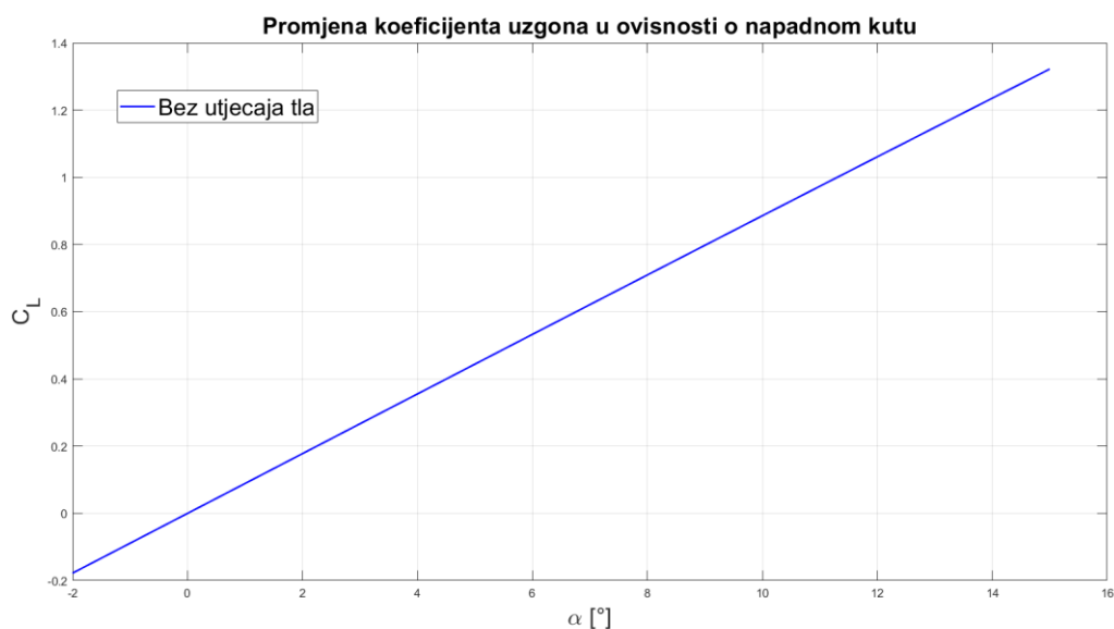
Slika 7 Promjena koeficijenta uzgona C_L u ovisnosti o napadnom kutu \alpha bez utjecaja tla
