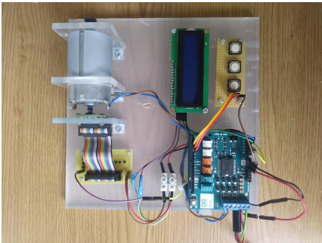
Slika 10. Eksperimentalni postav
