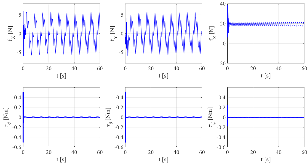
Slika 5.42: Upravljačke sile i momenti letjelice u zatvorenoj petlji AlgDRC uz prisustvo vanjskih poremećaja za drugi slučaj.
