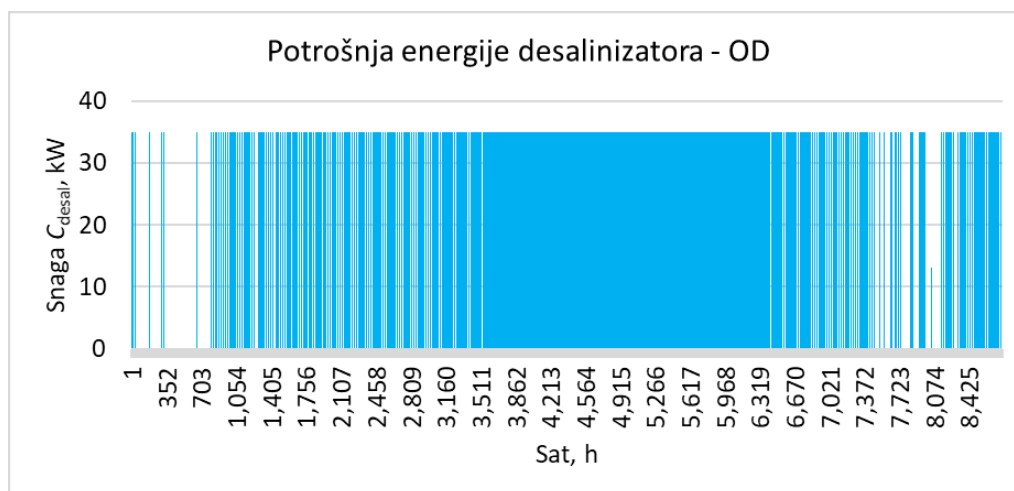
Slika 49. Dijagram potrošnje električne energije desalinizatora u OD scenariju
