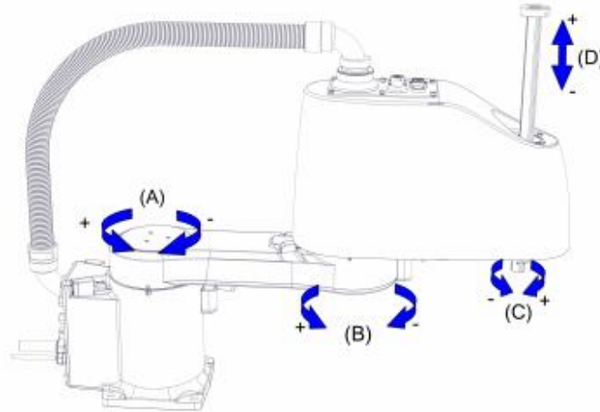
Slika 12 Prikaz stupnjeva slobode gibanja IRB 910SC SCARA manipulatora
