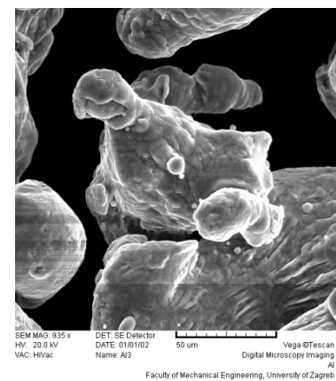
Slika 3.5 Prikaz oblika čestica praška Rototec 29220 dobivenih SEM mikroskopom.
