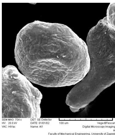
Slika 3.5 Prikaz oblika čestica praška Rototec 29220 dobivenih SEM mikroskopom.
