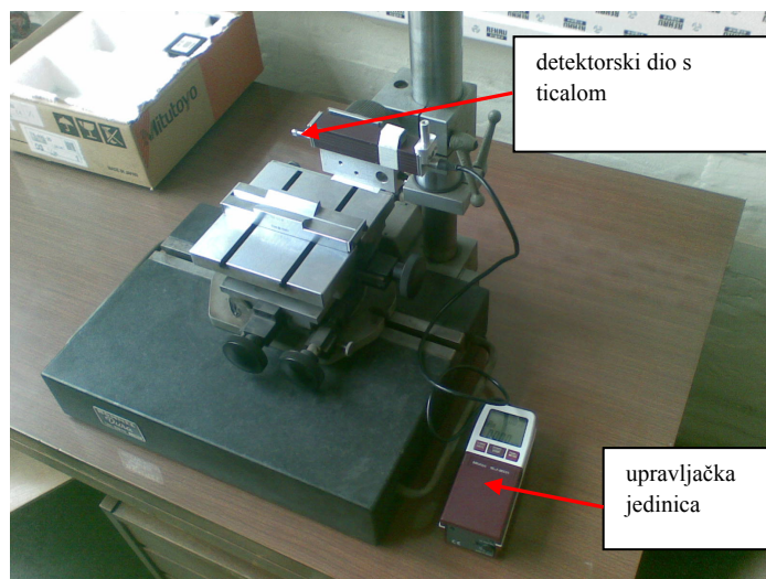
Slika 3.25 Uređaj s ticalom za 2D ispitivanje amplitudnih parametara hrapavosti.
