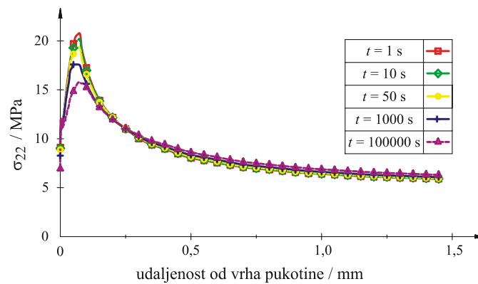
Slika 109. Relaksacija maksimalnog glavnog napreznja, \sigma_{22} , u ovisnosti o udaljenosti od vrha zarezha i vremenu puzanja
