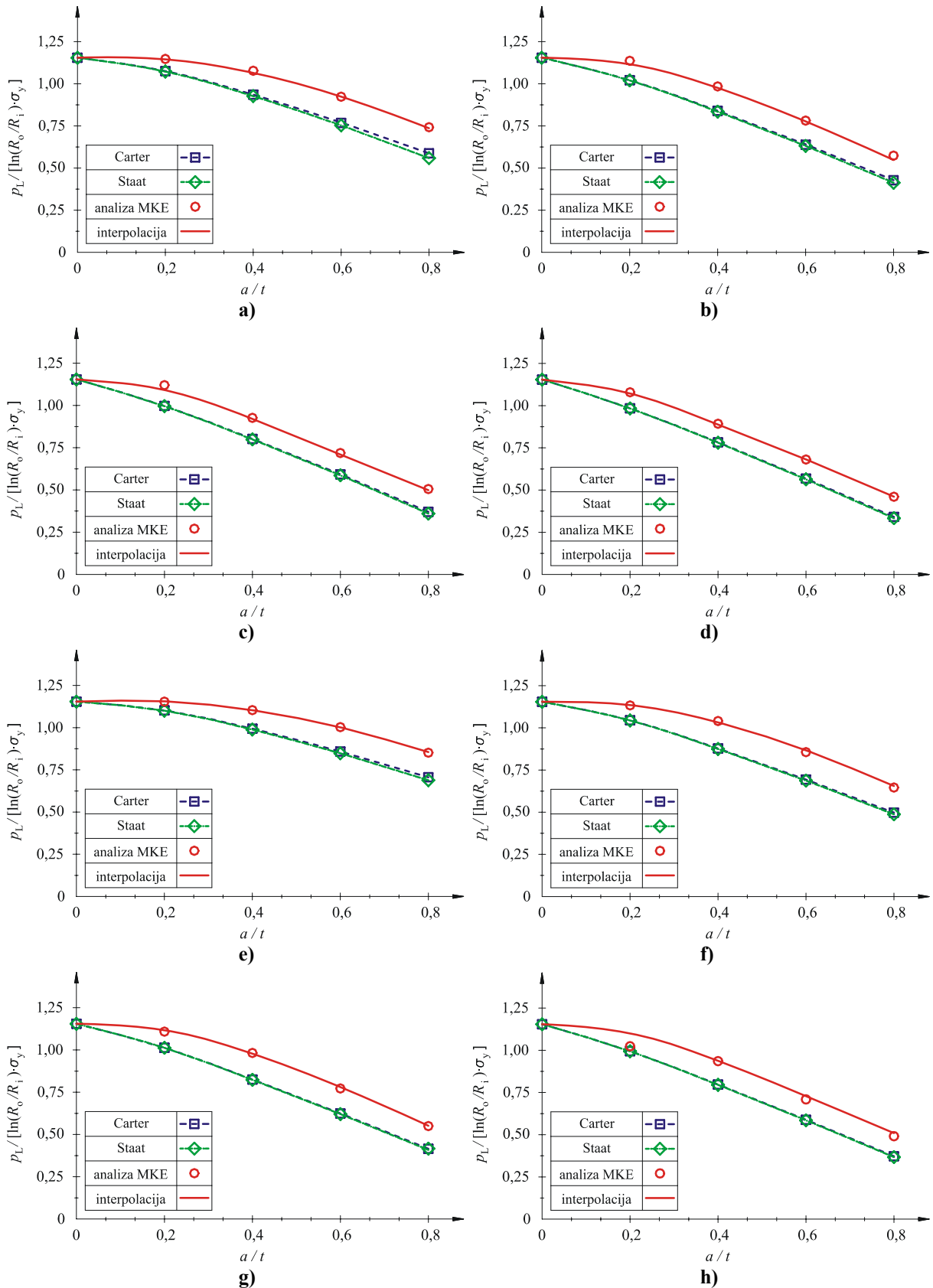
Slika 41. Usporedba graničnog tlaka za cijevi opterećene unutarnjim tlakom s vanjskom osnom polueliptičkom pukotinom s izrazima iz literature [21] i [20, 29] za: a) R_i/t = 4 i c/a = 5 ; b) R_i/t = 4 i c/a = 10 ; c) R_i/t = 4 i c/a = 15 ; d) R_i/t = 4 i c/a = 20 ; e) R_i/t = 10 i c/a = 5 ; f) R_i/t = 10 i c/a = 10 ; g) R_i/t = 10 i c/a = 15 i h) R_i/t = 10 i c/a = 20
