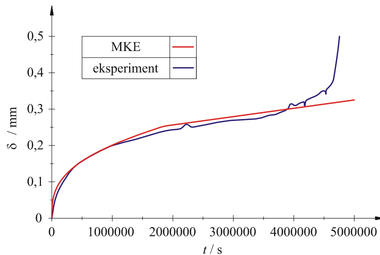
Slika 105. Usporedba dijagrama međusobne ovisnosti pomaka, \delta , točke A o vremenu puzanja, t , materijala pri 60°C i za \sigma_{\text{net}} = 8 MPa dobivenog eksperimentalno, Hamouda i ostali autori [33, 36, 37], i numerički primjenom korisničke rutine CREEP u programskom paketu ABAQUS
