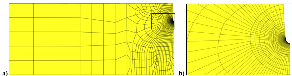
Slika 106. Deformirani oblik osnosimetrične epruvete s potpunim obodnim zarezom diskretizirane Mrežom 3: a) dio epruvete i b) područje oko vrha zarezova
