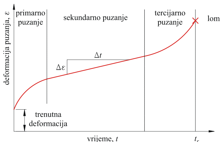
Slika 13. Dijagram puzanja konstrukcije opterećene konstantnim naprezanjem [52, 56]
