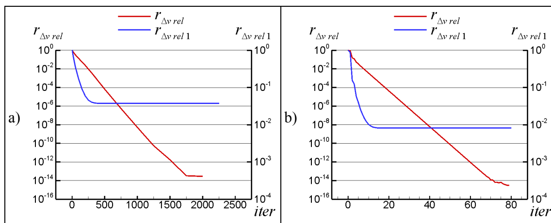
Slika 5.40 Primjer 8. Konvergencija rješenja prema srednjim relativnim razlikama brzine r_{\Delta v rel 1} i vlastitim r_{\Delta v rel} : a) SIMPLE; b) FLOP
