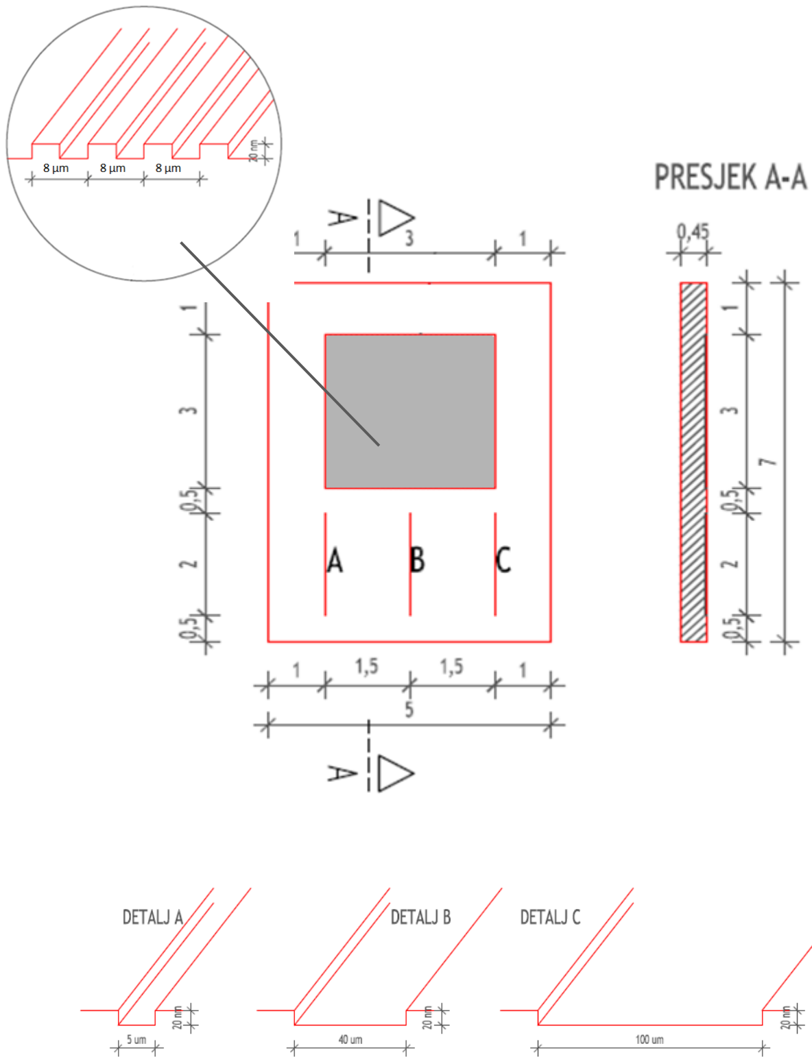
Slika 6.5 Model novog etalona
