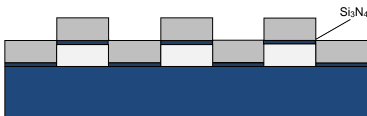
Slika 7.2 Presjek novog etalona
