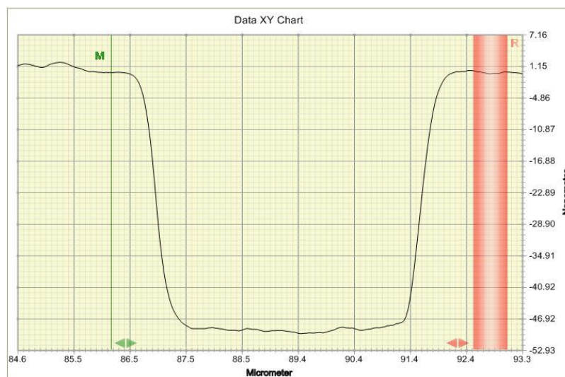
Slika 7.22 Brazde širine 5 \mu\text{m} na etalonu oznake REH 50/2
