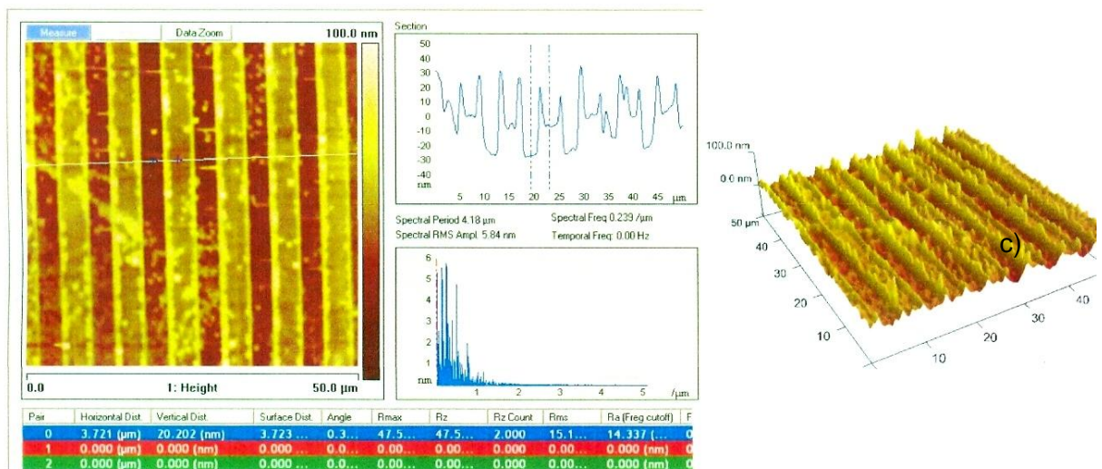
Slika 7.10 a) 2D prikaz etalona oznake REH 20/1 snimljenog AFM-om nakon prevlačenja b) Profili na snimljenom etalonu c) 3D prikaz etalona
