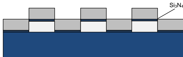
Slika 7.2 Presjek novog etalona
