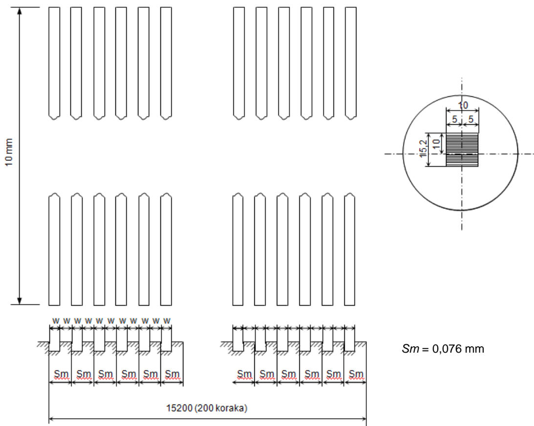
Slika 4.5 Mjerna površina sa slijedom pravokutnih brazdi
