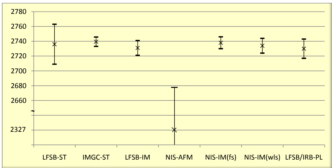
Slika 5.12 Rezultati usporedbenih mjerenja za dubinu brazde nazivno 2700 nm
