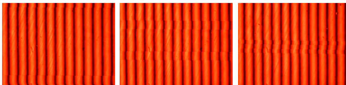
Slika 7.12 a) Interferogram na etalonu oznake REH 20/1- brazda širine 100 \mu\text{m} b) Interferogram na etalonu oznake REH 20/1- brazda širine 40 \mu\text{m} c) Interferogram na etalonu oznake REH 20/1- brazda širine 5 \mu\text{m}
