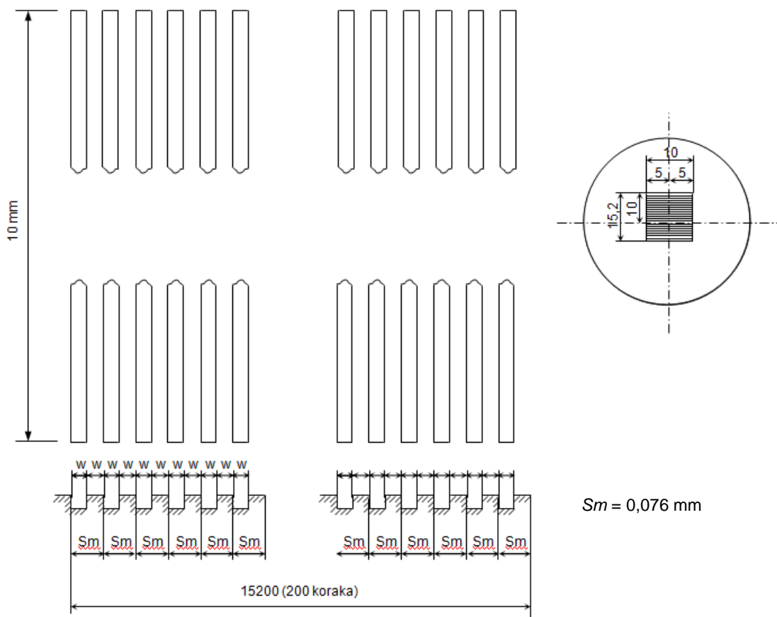
Slika 4.5 Mjerna površina sa slijedom pravokutnih brazdi
