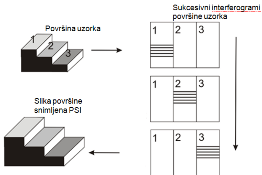
Slika 3.15 Princip PSI
