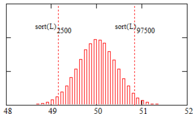
Slika 8.7 Funkcije gustoće vjerojatnosti g(d) za etalon nazivne dubine brazde 50 nm
