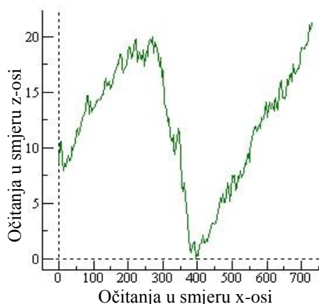
Slika 7.25 Profil brazde snimljen STM-om
