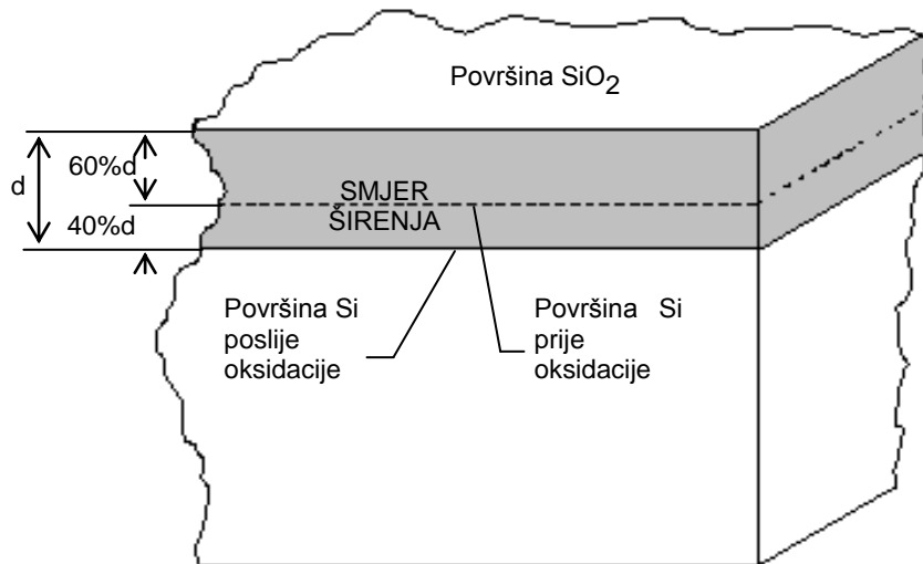
Slika 6.1 Formiranje sloja SiO 2 na Si pločici
