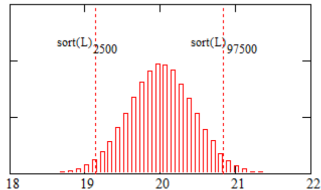
Slika 8.6 Funkcije gustoće vjerojatnosti g(d) za etalon nazivne dubine brazde 20 nm
