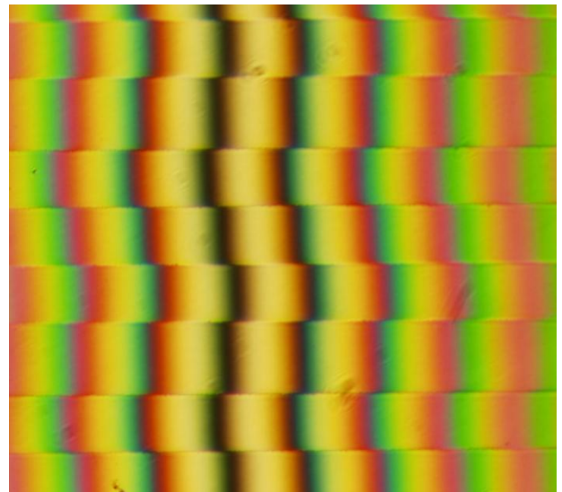
Slika 6.19 Etalon nazivne dubine brazde 50 nm. Interferogram na površini prevučenoj kromom
