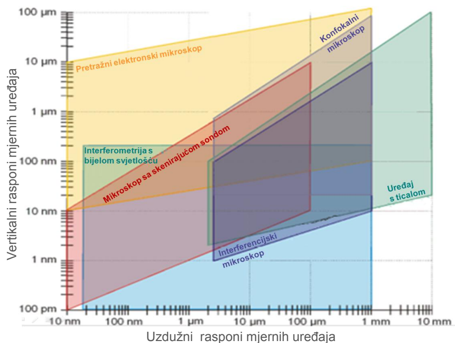
Slika 2.1 Mjerna područja uređaja u mikro- i nanomjeriteljstvu
