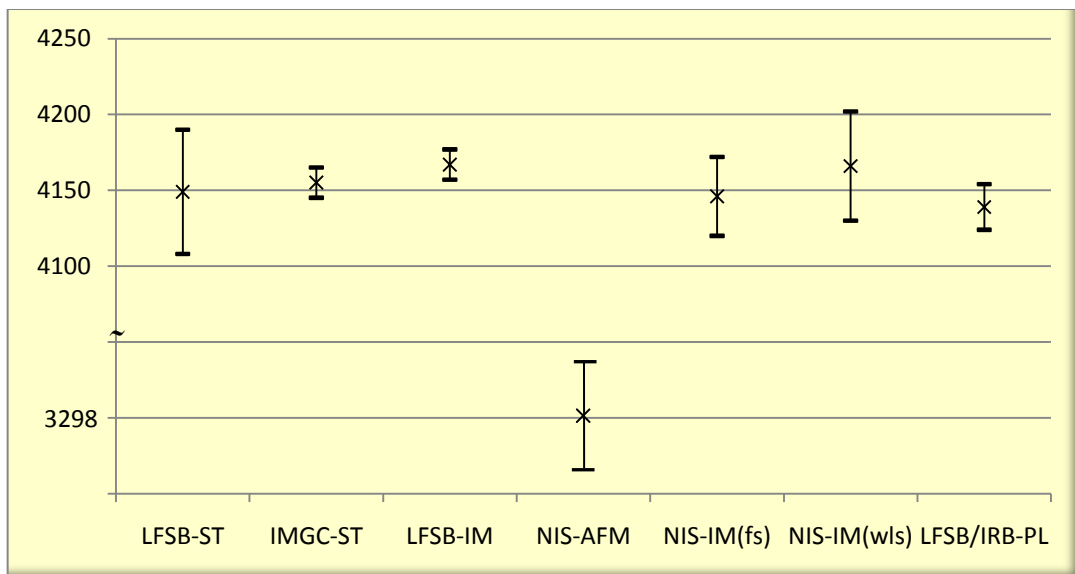
Slika 5.13 Rezultati usporedbenih mjerenja za dubinu brazde nazivno 4100 nm
