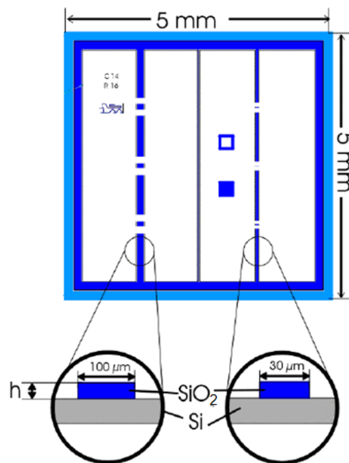
Slika 5.15 Prikaz etalona mjenenog u NANO 2 interkomparaciji
