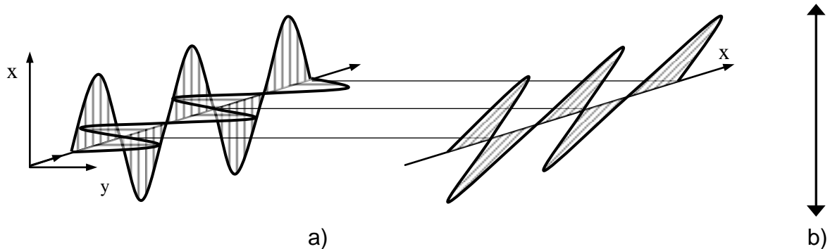
Slika 3.17 a) Ortogonalni međusobno koherentni linearno polarizirani valovi i rezultantni linearno polarizirani val zakrenute ravnine vibracije. b) Uobičajeni način prikazivanja linearno polariziranog vala.
