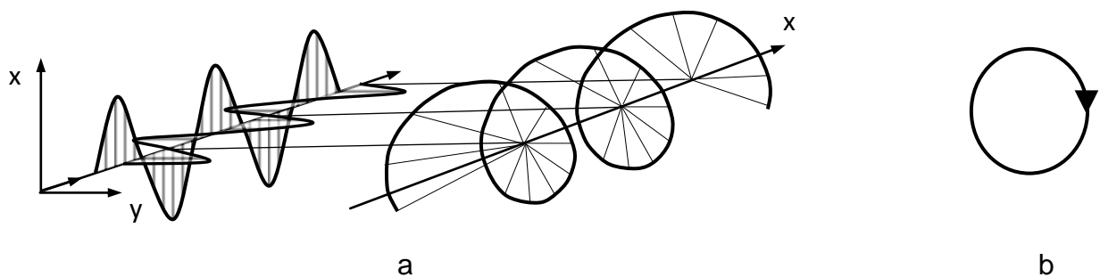
Slika 3.18 a) Ortogonalni linearno polarizirani valovi jednakih amplituda pomaknuti u fazi za \lambda/4 i rezultantni kružno polarizirani val. b) Uobičajeni način prikazivanja kružno polariziranog vala.
