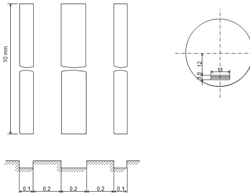
Slika 4.4 Mjerna površina s tri široke brazde
