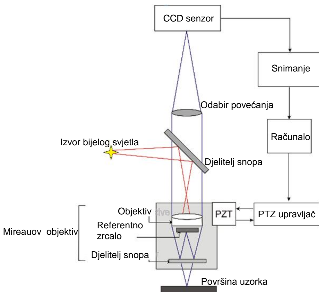
Slika 3.14 Konfiguracija VLS interferencijskog sustava
