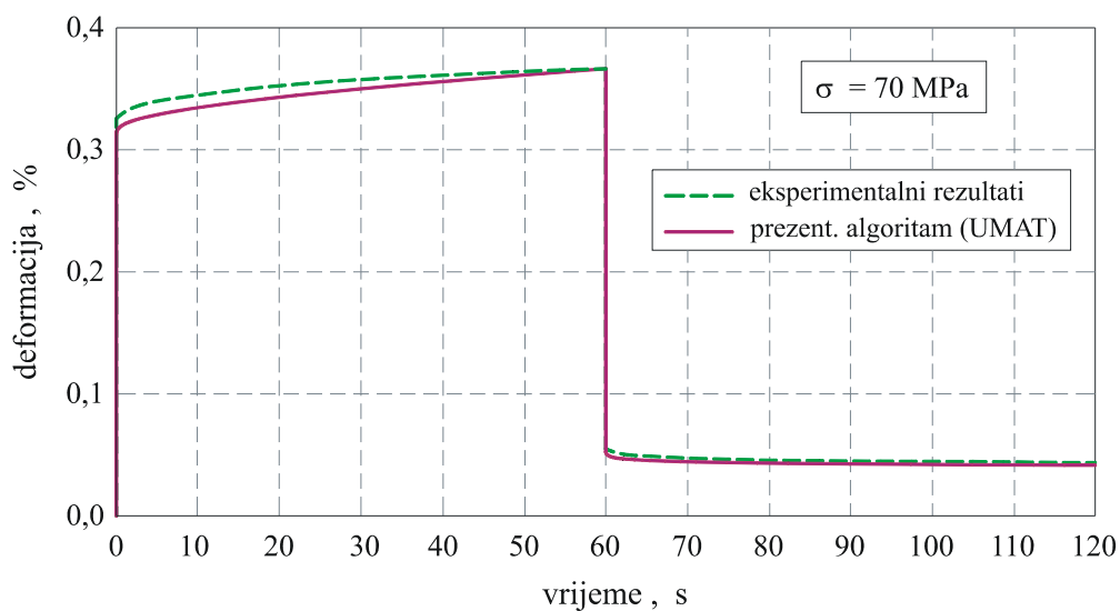
Slika 73. Usporedba numeričkih i eksperimentalnih vrijednosti ovisnosti deformacije o vremenu za goveđe kortikalno koštano tkivo pri naprežanju od 70 MPa
