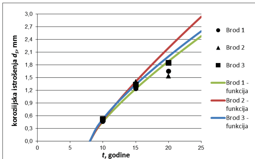
Slika 2.19 - Izmjerena i predviđena srednja vrijednost korozijskog istrošenja uzdužnjaka palube tankova tereta
