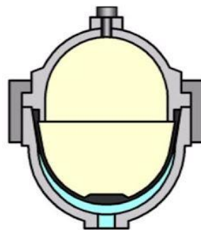
Slika 2. Membranski akumulator
