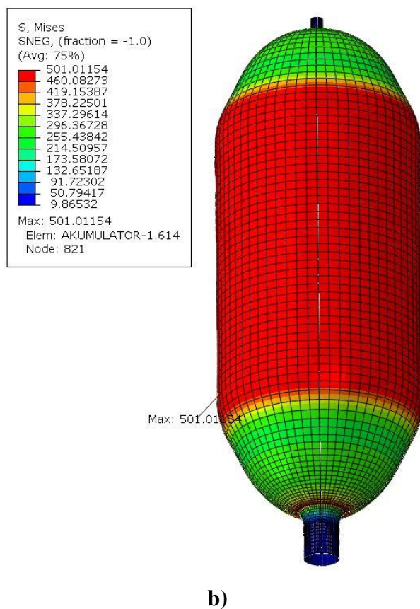
Slika 45. Raspodjela ekvivalentnog napreznja prema von Misesu (u MPa) za model diskretiziran sa a) 15726, b) 1410 elemenata oznake S8R5
